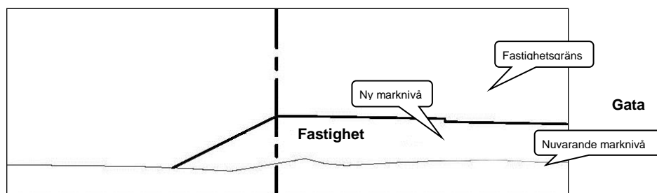
Sektion med illustration av slänt i form av utfyllnad på fastighet.
