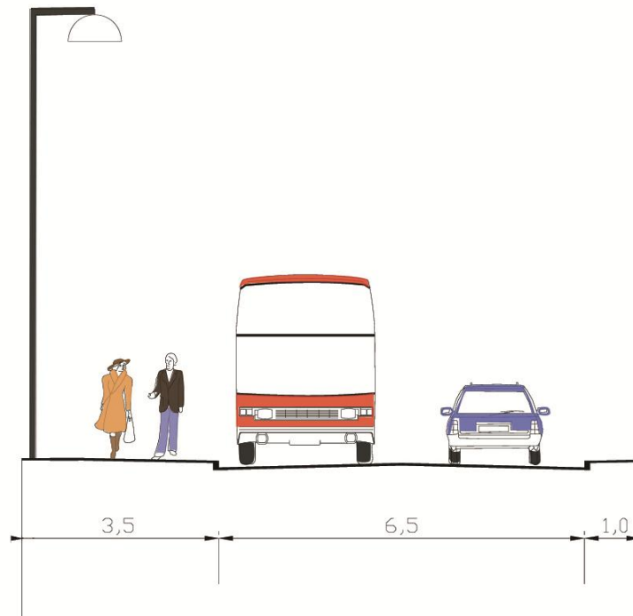
Vägsektion huvudgata för buss.
