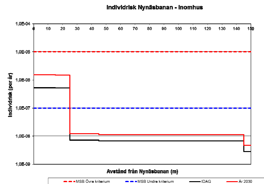
Figur 5.2. Individrisk inomhus utmed Nynäsbanan i höjd med planområdet del av Bonden 1 och del av Hammartorp 1:1 m.fl. i Trångsund. (Observera att frekvensen redovisas med logaritmisk skala.)
