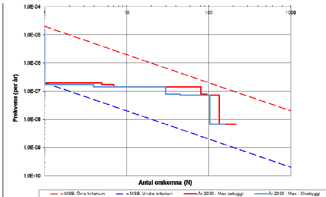
Figur 5.3. F/N-kurva som redovisar samhällsrisknivån för ny bebyggelse respektive befintliga förutsättningar inom del av Bonden 1 och del av Hammartorp 1:1 m.fl. och dess närmaste omgivning med avseende på olycksrisker förknippade med trafiken på Nynäsbanan. (Observera att frekvensen redovisas med logaritmisk skala.)
