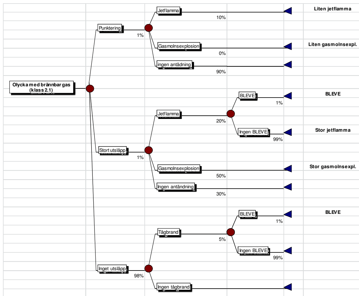
Figur A.1. Händelsetråd olycka med transport av brännbar gas (klass 2.1).
