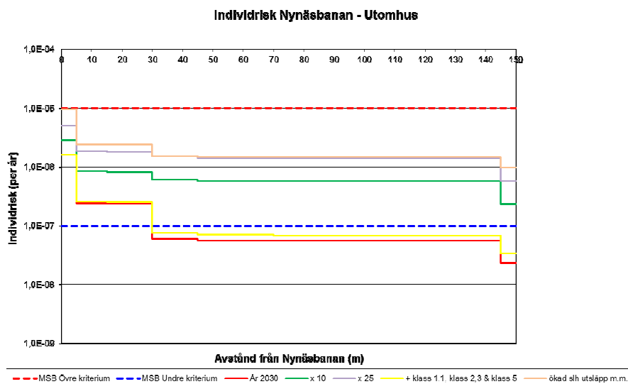
Figur 5.4. Känslighetsanalys – Individerisk utomhus . (Observera att frekvensen redovisas med logaritmisk skala.)
