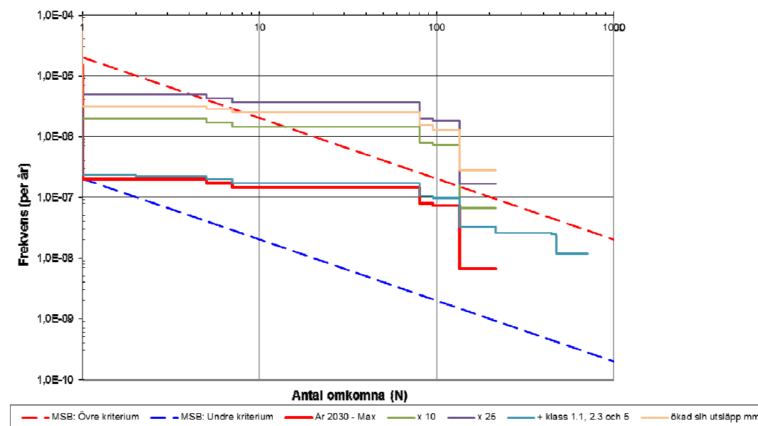
Figur 5.6. Känslighetsanalys – Samhällsrisk. (Observera att frekvensen redovisas med logaritmisk skala.)
