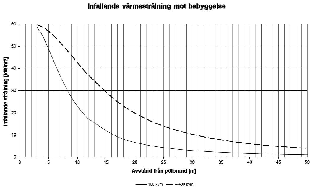
Figur B.3. Infallande strålning som funktion av avståndet från pölbrand.
