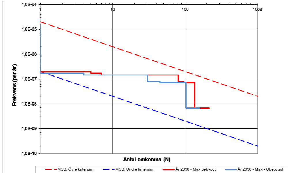
Figur C.5. F/N-kurva som redovisar samhällsrisknivån för ny bebyggelse respektive befintliga förutsättningar inom del av Bonden 1 och del av Hammartorp 1:1 m.fl. och dess omgivning med avseende på olycksrisker förknippade med trafiken på Nynäsbanan.
