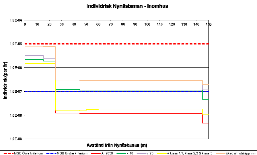
Figur 5.5 Känslighetsanalys – Individerisk inomhus . (Observera att frekvensen redovisas med logaritmisk skala.)
