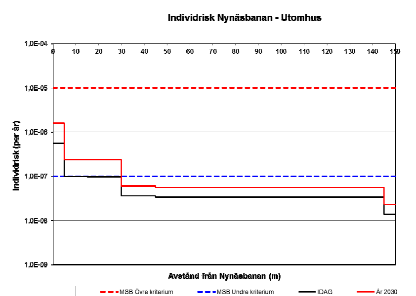
Figur 5.1. Individrisk utomhus utmed Nynäsbanan i höjd med planområdet del av Bonden 1 och del av Hammartorp 1:1 m.fl. i Trångsund. (Observera att frekvensen redovisas med logaritmisk skala.)
