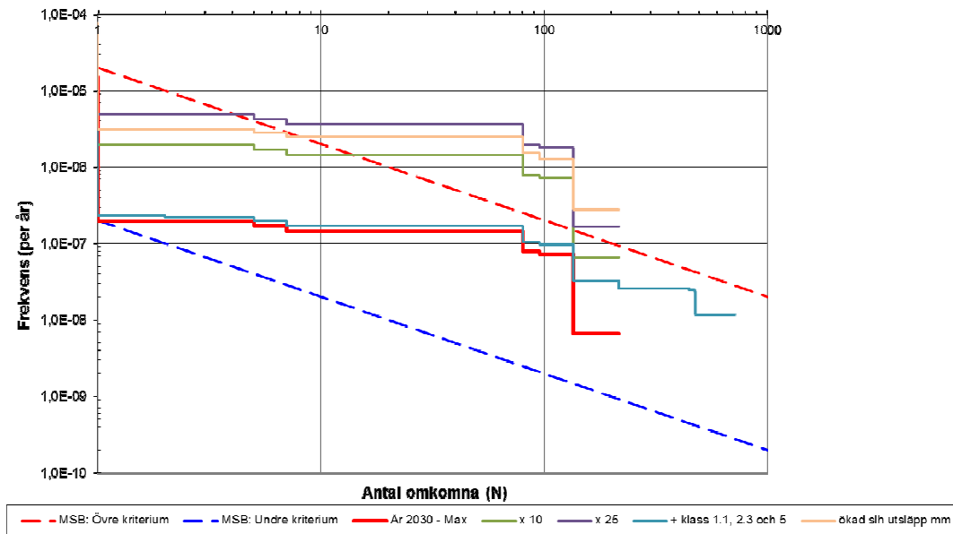
Figur C.6. Känslighetsanalys – Samhällsrisk.
