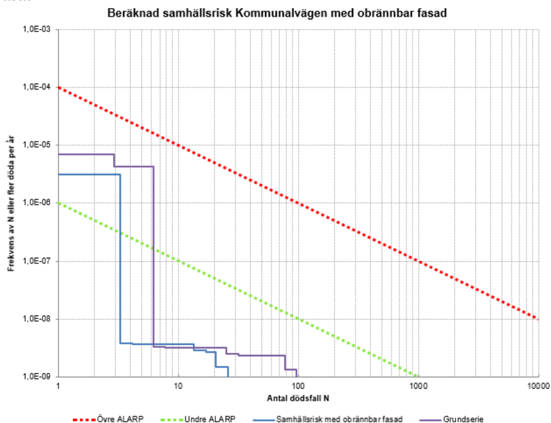
Figur 12. Grov uppskattning av samhällsrisknivå med obännbar fasad.
