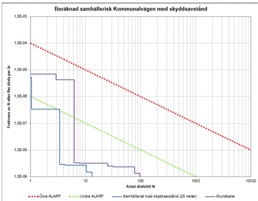
Figur 13 Grov uppskattning av samhällsrisknivå med åtgärden skyddsavstånd.
