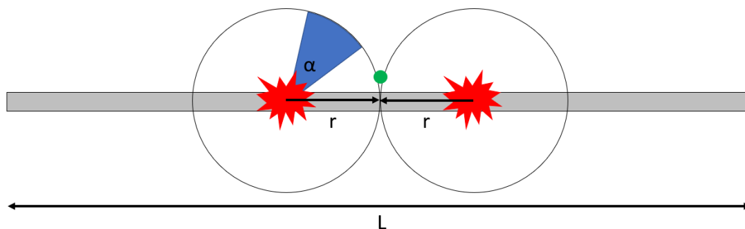
Figur 21. Sannolikheten att en person (markerad i grönt) precis intill en farligt gods led påverkas av en olycka med konsekvensavstånd r och spridningsvinkel \alpha .
