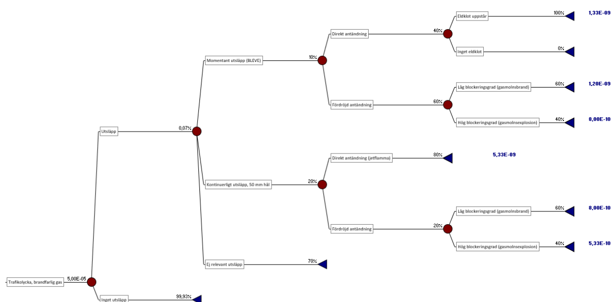
Figur A2. Händelseträd för brandfarlig gas. Frekvenser för olika händelser redovisas i slutet av händelseträdet (per år).
