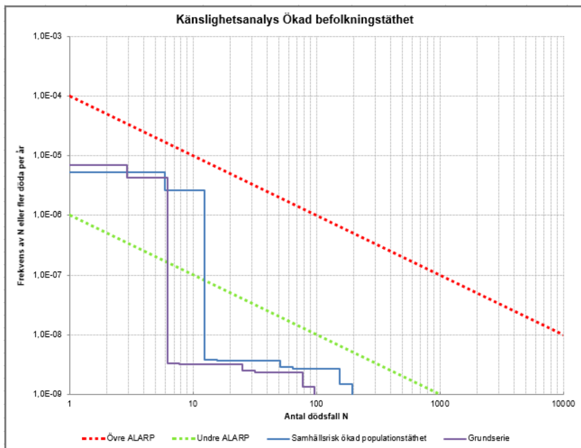
Figur 10. Beräknad samhällsrisk med 50 % ökad befolkningstäthet runt transportleden.
