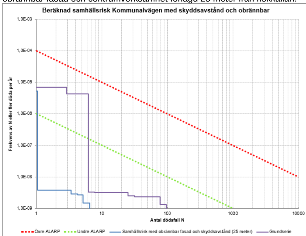
Figur 15 Grov uppskattning av samhällsriskenivå med obrännbar fasad och skyddsavstånd.
