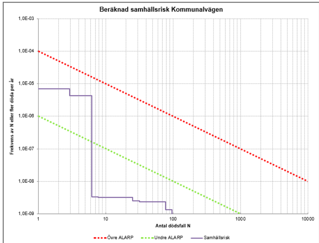
Figur 9. Beräknad samhällsrisk runt transportleden.
