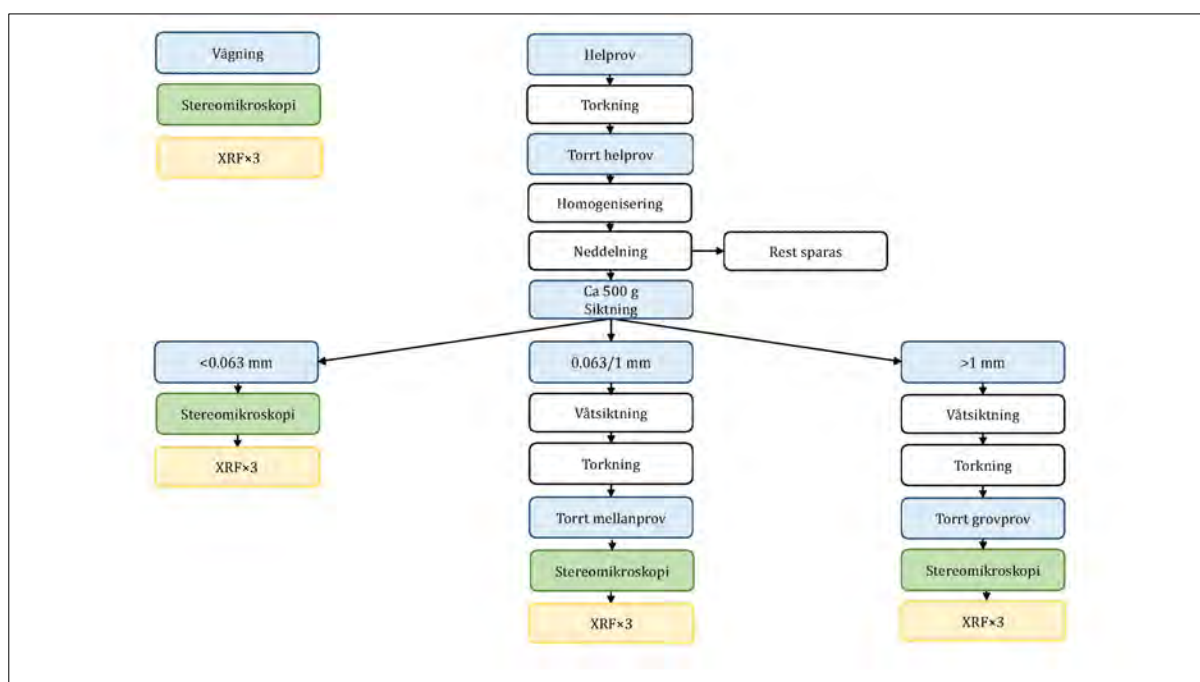
Figur 5. Schematisk bild över provberednings- och provbehandlingsförfarandet.
