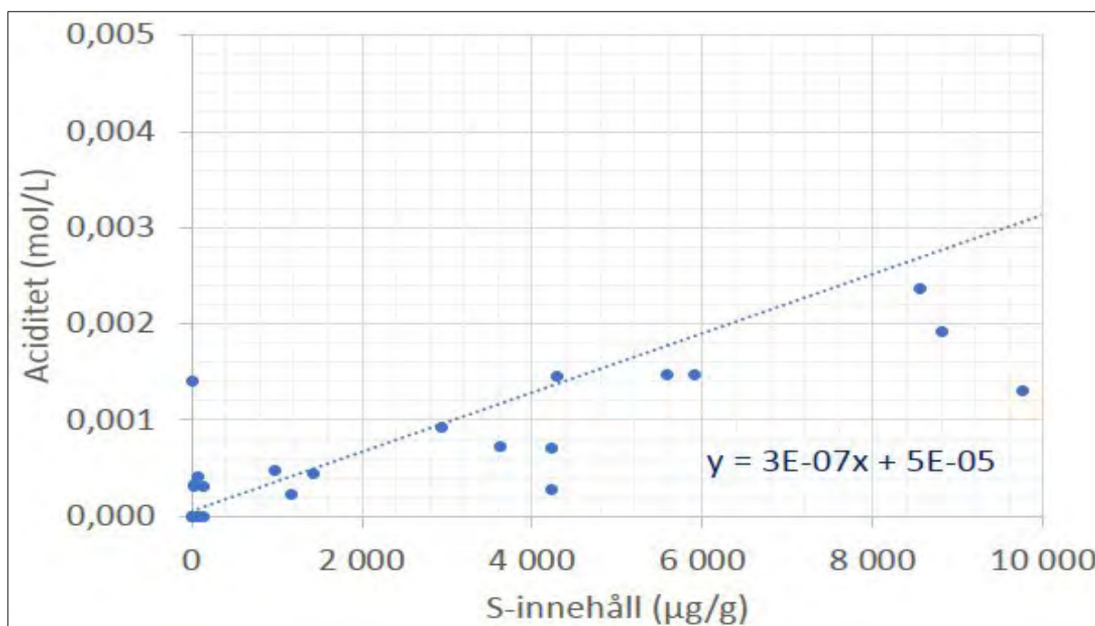
Figur 10. Finfraktionens potentiella försurningsförmåga uttryckt som samband mellan svavelhalt och försurningspotential (aciditet).
