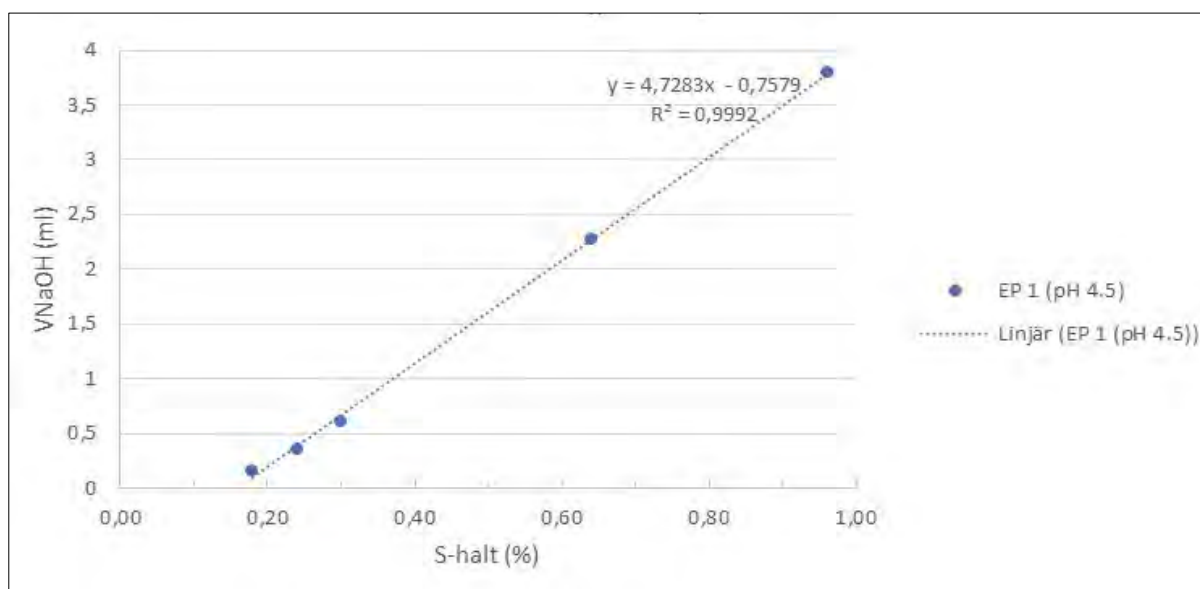
Figur 9. Korrelation mellan svavelhalt och volym av neutraliserande natriumhydroxid (NaOH) i BP10.
