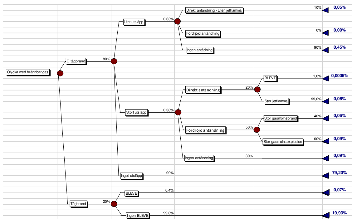
Figur A.2. Händelsetråd olycka med transport av brännbara gaser.
