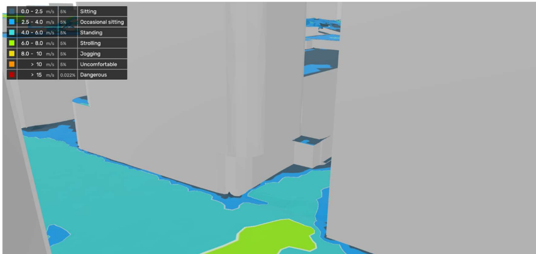
Figur 46. Vindkomfort baserad på årlig vindstatistik – Centralmarkens ingång.
