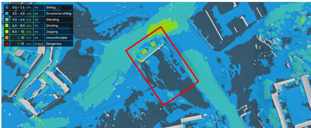
Figur 23: Vindkomfort – kvartal 3 (juli till september).
