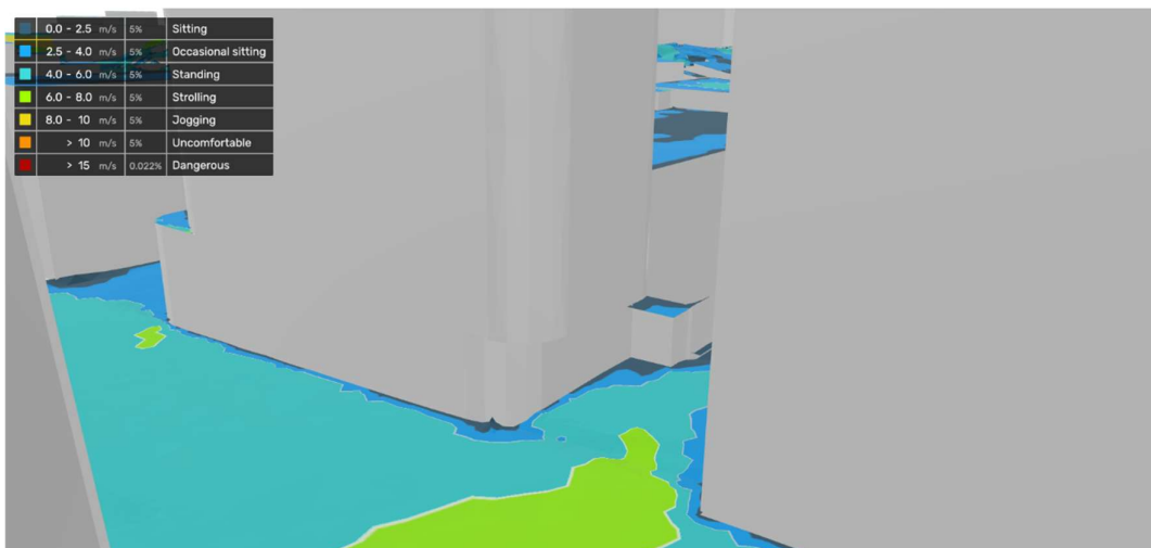
Figur 47. Vindkomfort - kvartal 1 (januari till mars).
