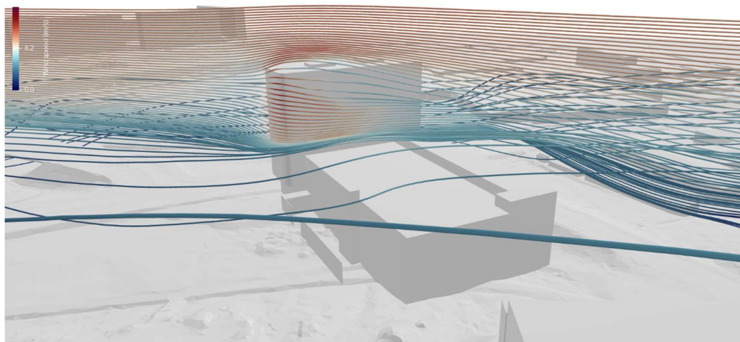
Figur 27. Strömlinjer för västliga vindar som visar hur vindflödet interagerar med Centralmarken.
