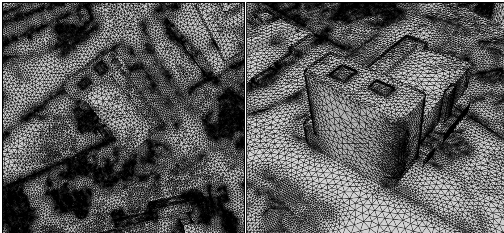
Figur 15: Mesh som använts till sydvästliga vindar – Skede 1.
