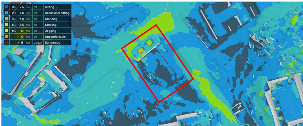
Figur 20: Vindkomfort baserad på årlig vindstatistik.
