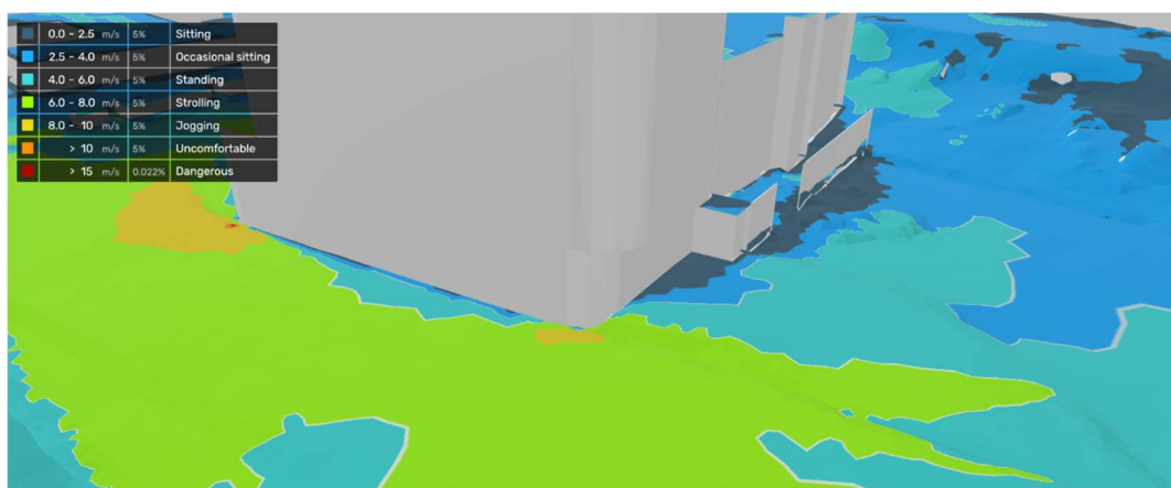
Figur 30. Vindkomfort - kvartal 4 (oktober till december).
