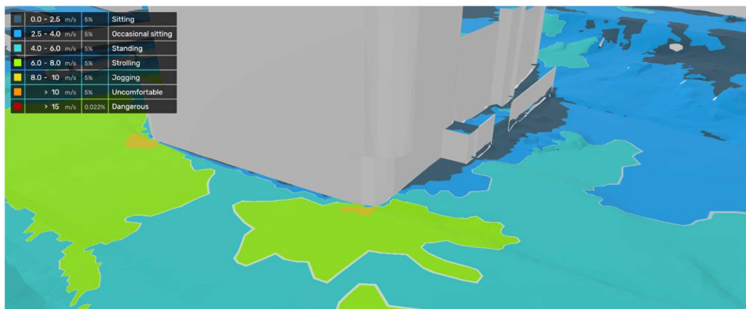
Figur 29. Vindkomfort baserad på årlig vindstatistik – Centralmarkens ingång.
