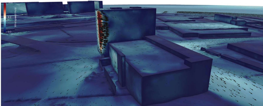
Figur 26. Vindhastigheter baserat på västliga vindar.
