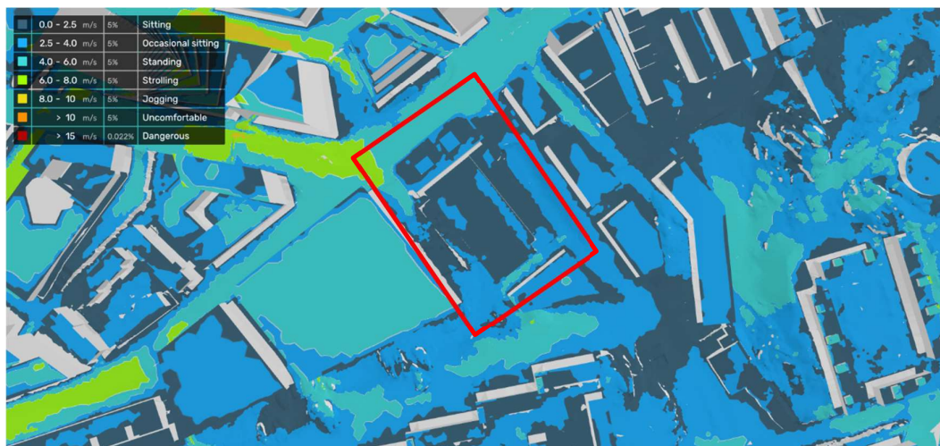
Figur 39: Vindkomfort baserad på årlig vindstatistik.
