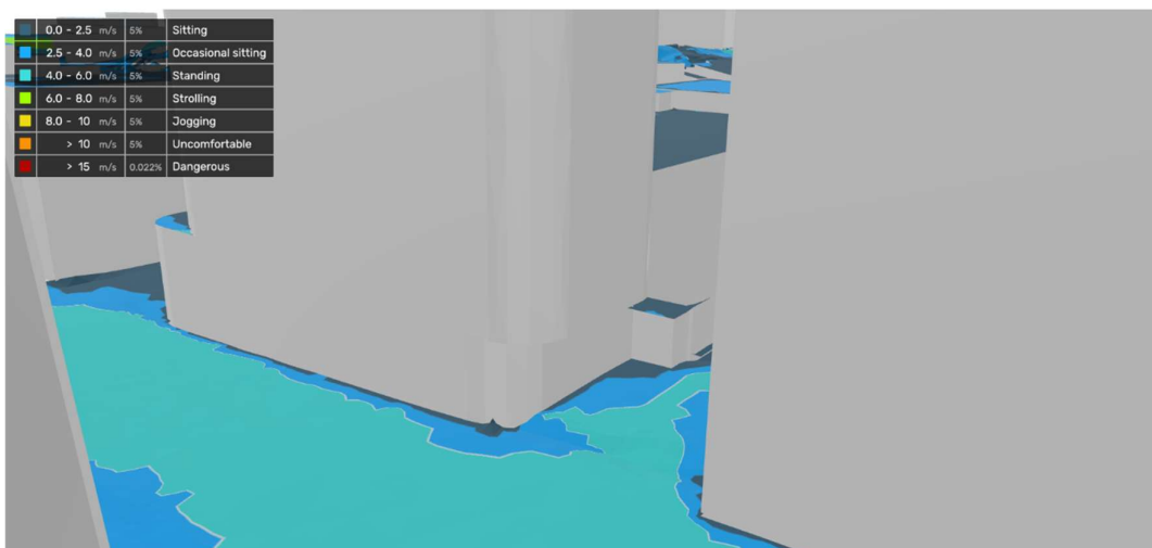
Figur 49. Vindkomfort - kvartal 3 (juli till september).
