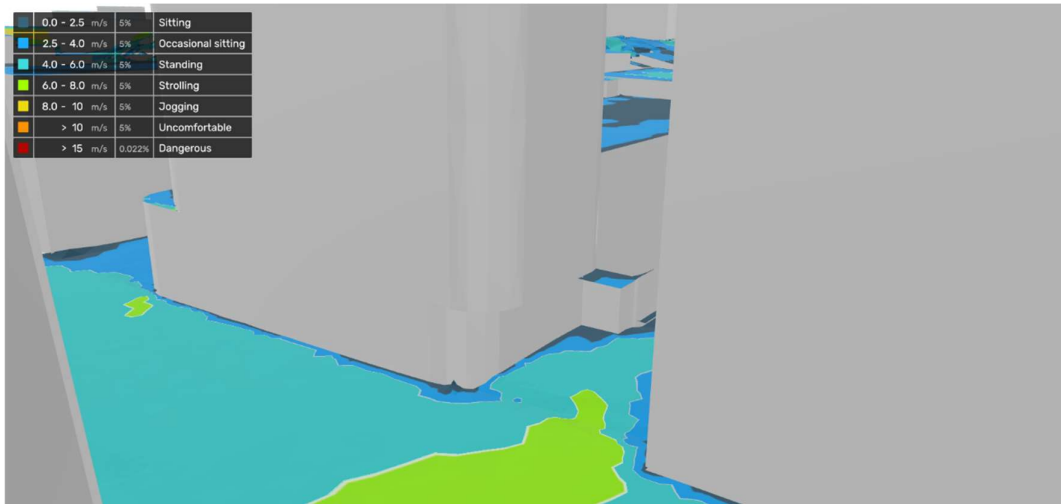
Figur 50. Vindkomfort - kvartal 4 (oktober till december).
