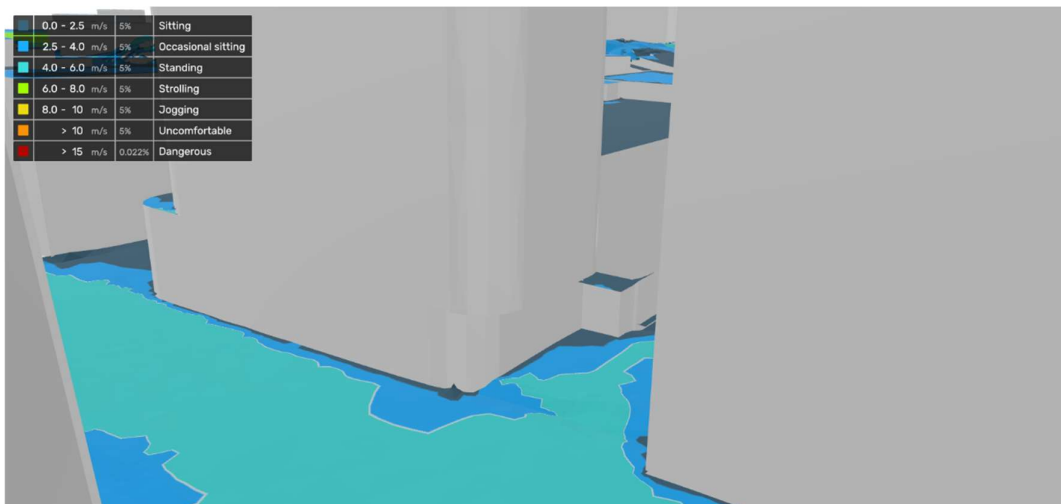
Figur 48. Vindkomfort – kvartal 2 (April till juni)
