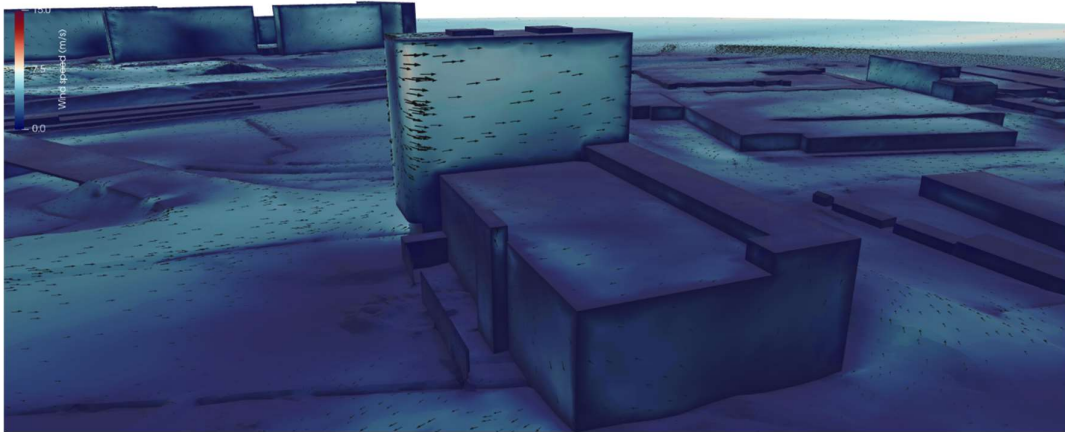
Figur 25. Vindhastigheter baserat på sydvästliga vindar.
