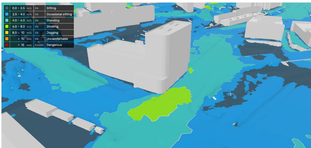
Figur 35. Lawsons vindkomfortskriterier – Q3 (juli – september).
