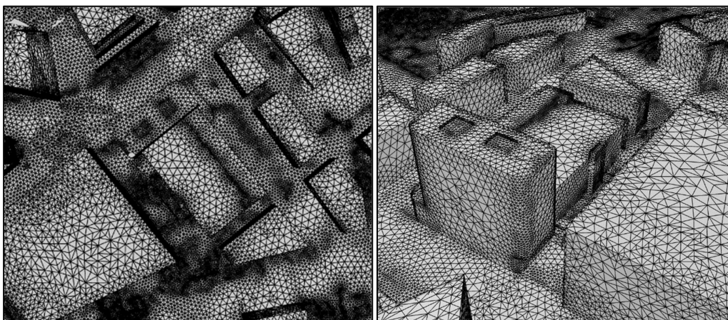
Figur 16: Beräkningsnät som använts till sydvästliga vindar – Skede 2.
