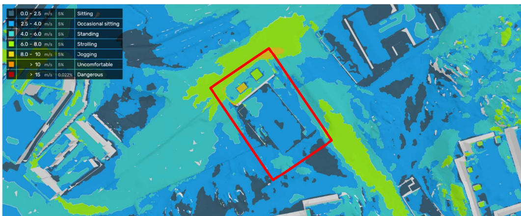
Figur 24: Vindkomfort – kvartal 4 (oktober till december).
