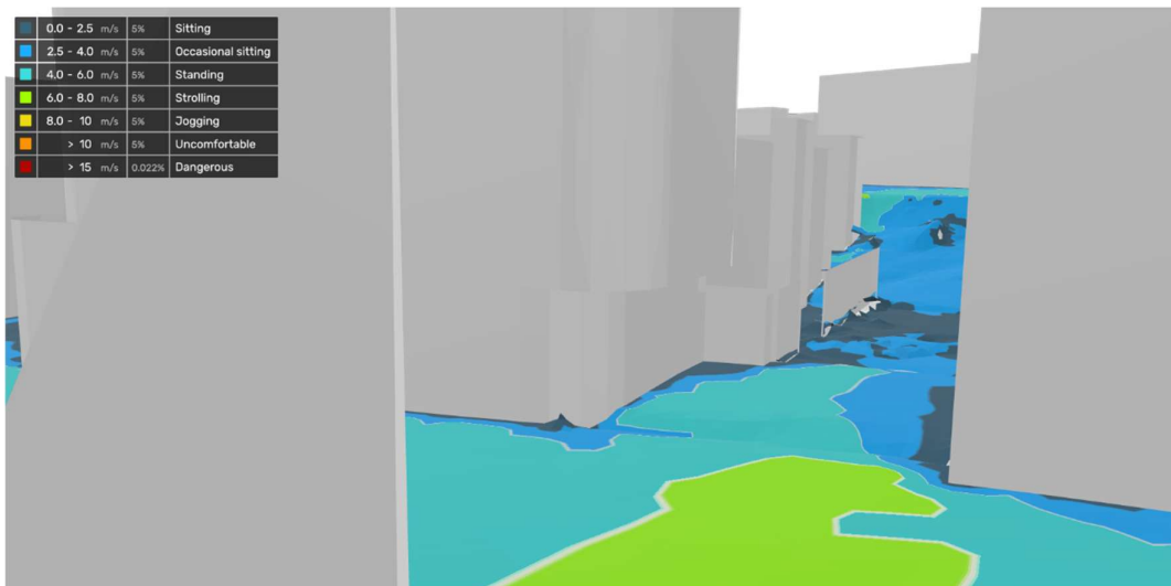
Figur 52. Vindkomfort baserad på årlig vindstatistik – lokalgatan.
