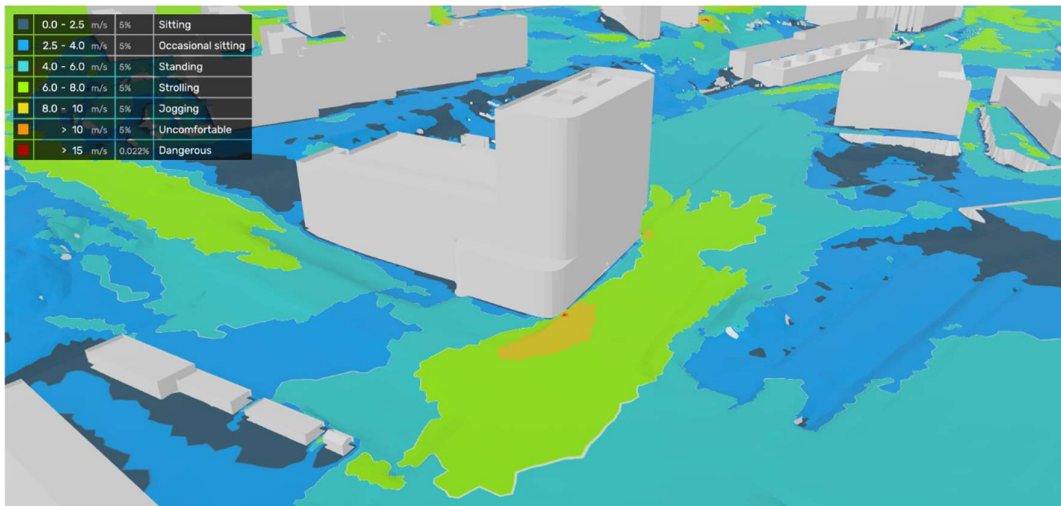
Figur 34. Lawsons vindkomfortskriterier – Q4 (oktober – december).
