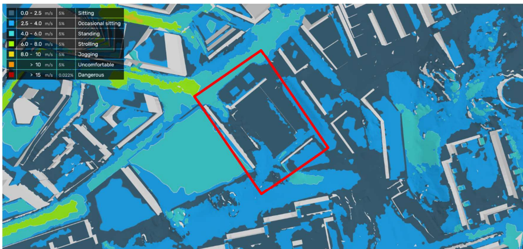
Figur 42: Vindkomfort – kvartal 3 (juli till september).
