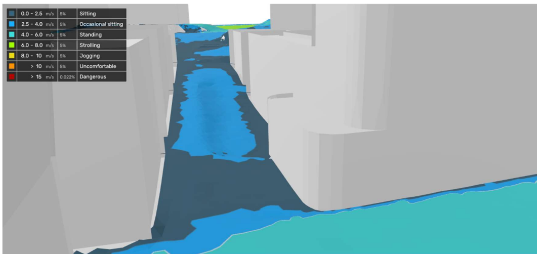
Figur 55. Vindkomfort - kvartal 3 (juli till september).
