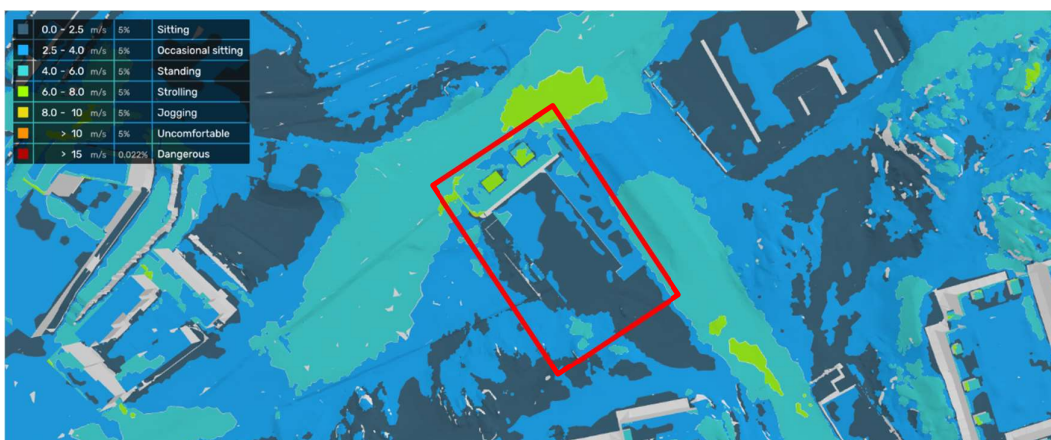
Figur 22: Vindkomfort – kvartal 2 (april till juni).
