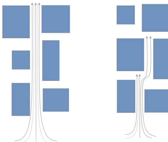
Figur 4. Venturieffekten (vänster) och vindblockeringseffekten (höger).
