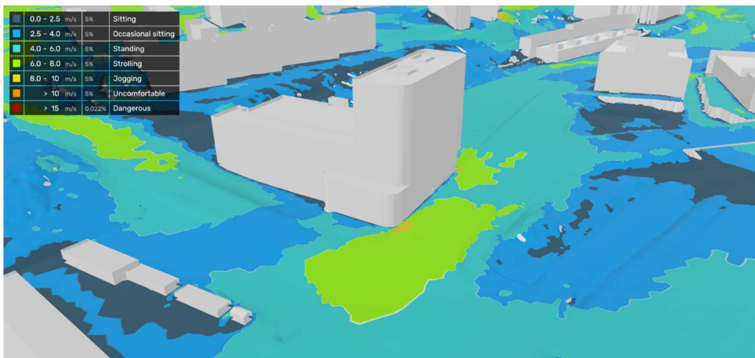
Figur 33. Lawsons vindkomfortskriterier – årsmedel
