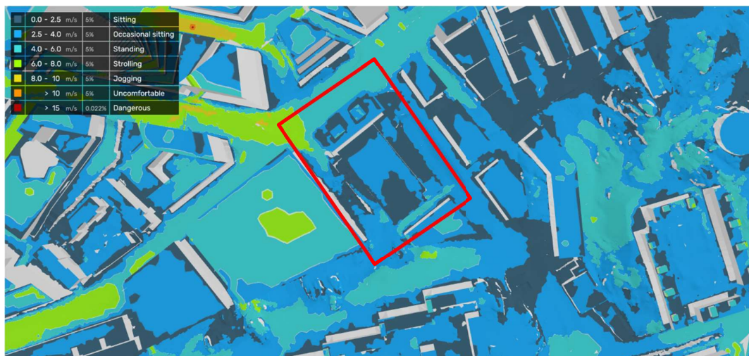
Figur 43: Vindkomfort – kvartal 4 (oktober till december).
