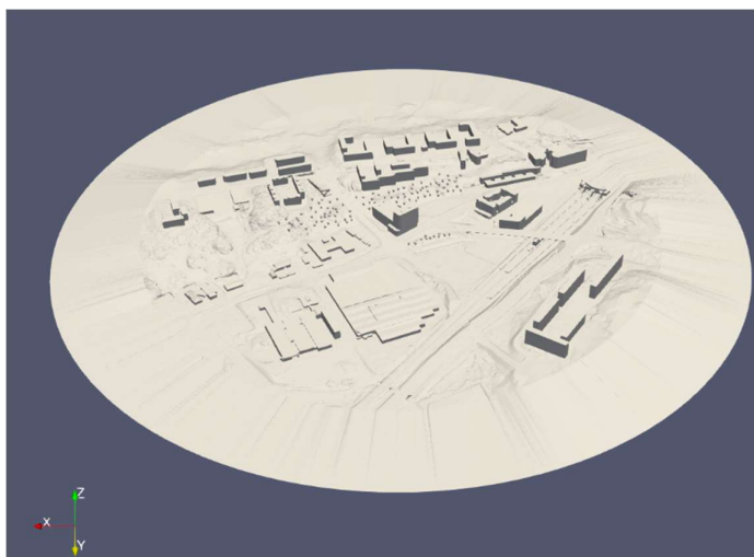
Figur 1. Modell som använts för simulering av Skede 1.
