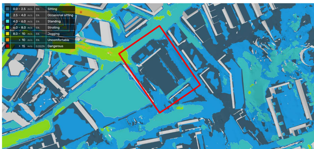
Figur 40: Vindkomfort – kvartal 1 (januari till mars).
