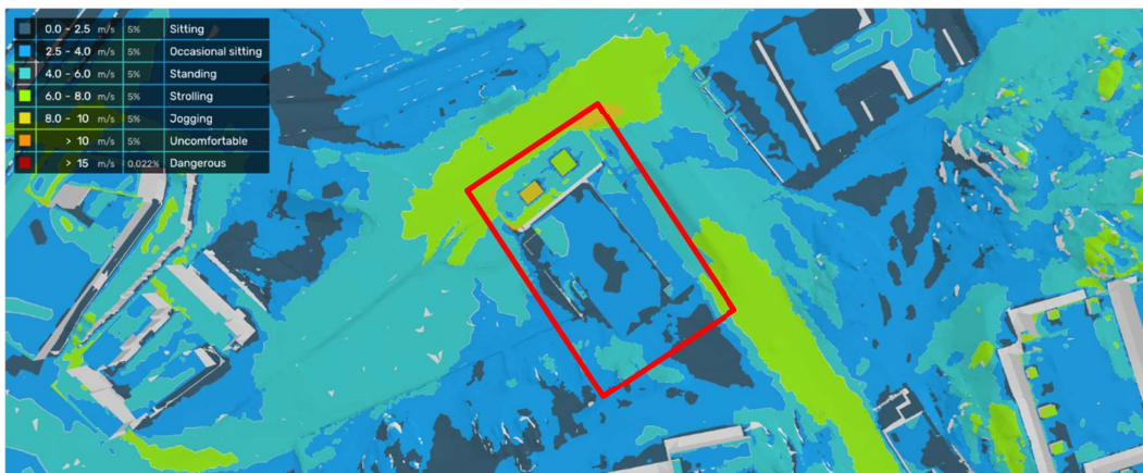
Figur 21: Vindkomfort – kvartal 1 (januari till mars).
