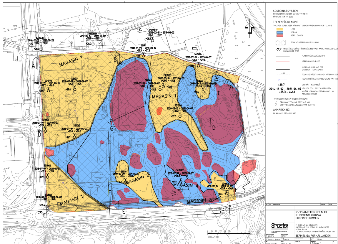
Figur 15. Befintliga grundvattenförhållanden (Structor Geoteknik, 2021)
