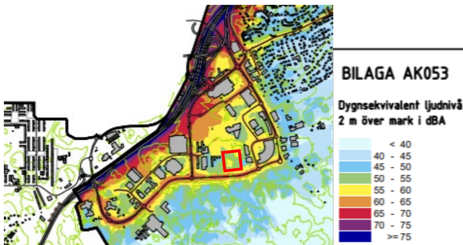
Figur 28. Dygnsekvivalent ljudnivå 2 m över mark i dBA. Källa: Kommunens bullerkartläggning, Tyréns, 2014, bilaga AK05 Dygnsekvivalent ljudnivå, Alla vägar, höjd 2m, del ett (nya hastigheter). Aktuellt område ungefärligt markerat med röda linjer.
