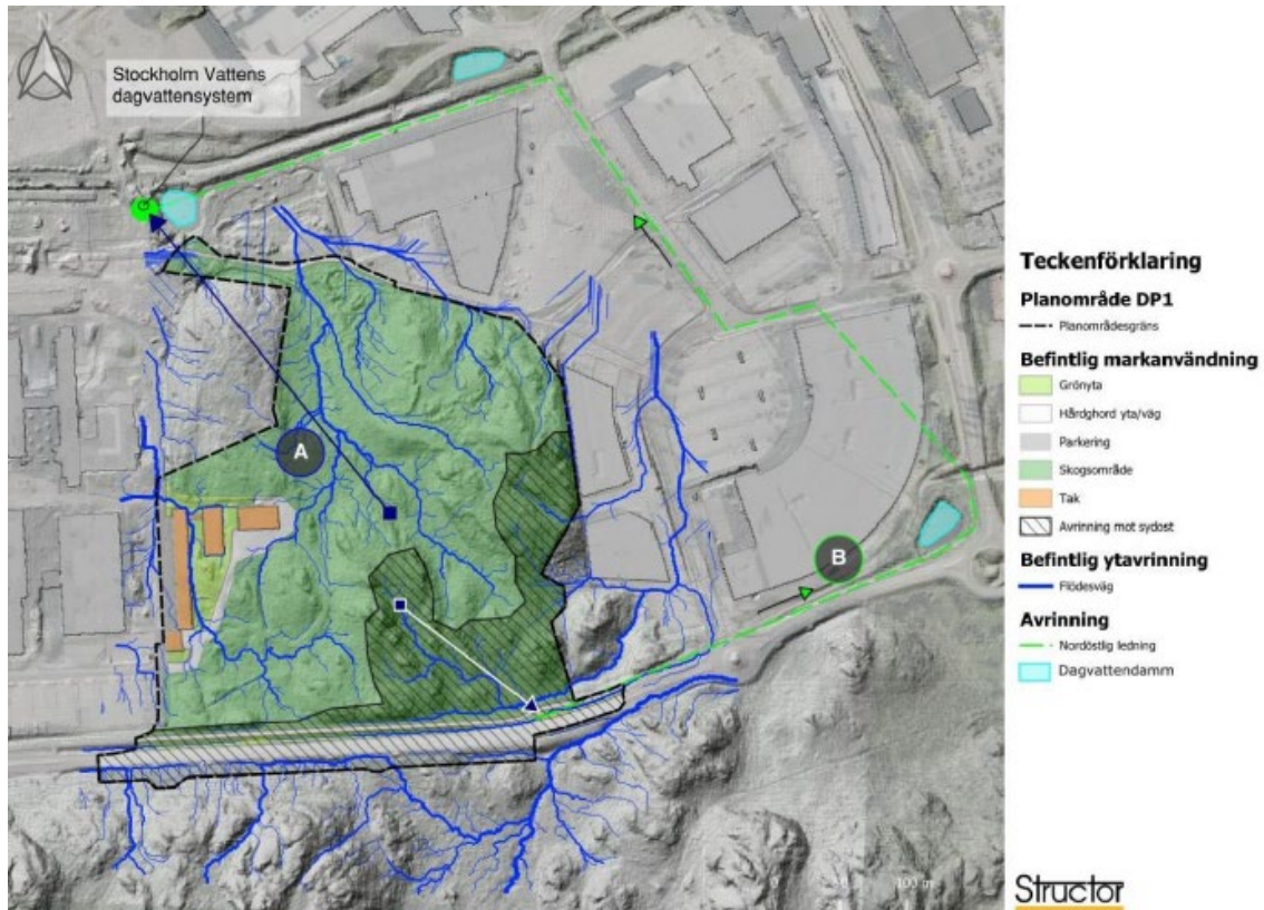
Figur 18. Avrinning i befintlig situation, tolkad efter grundkarta. Detaljplaneområdet är markerat med en svart polygon. Avrinningens riktning visas med blå och gröna flödespilar. Det östra avrinningsområdet med avrinning i sydöstlig riktning är markerat med skraffering (Structor Vatten och Miljö, 2021, reviderad 2024).
