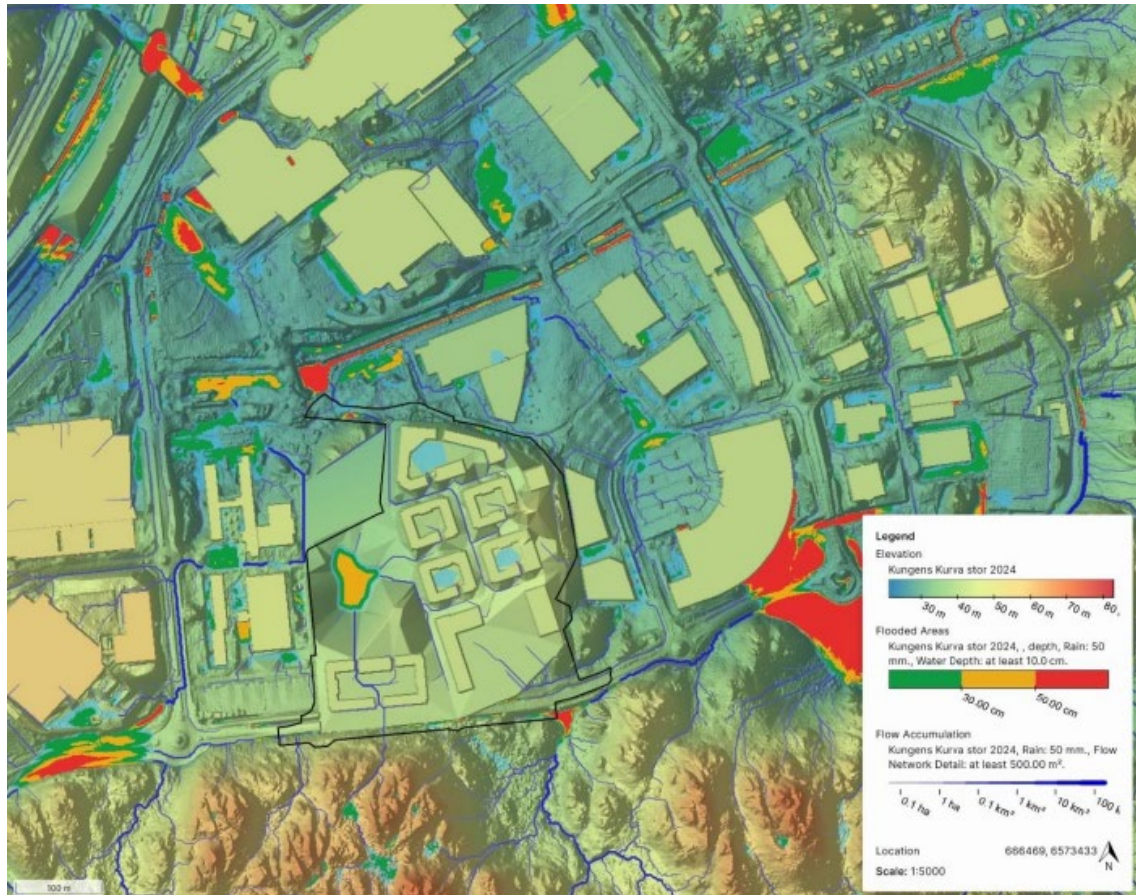
Figur 20. Skyfallsanalys för planförslaget inom och i anslutning till planområdet vid 50 mm nederbörd. Färgade områden visar instängda områden/lågpunkter där vatten kommer ansamlas och blåa linjer visar sekundära avrinningsvägar. Gröna områden visar ett vattendjup på 0–30 cm, gula områden 30–50 cm och röda områden visar vattendjup större än 50 cm. Detaljplaneområdesgräns redovisas med en svart polygon. (Structor Vatten och Miljö, 2021, reviderad 2024).
