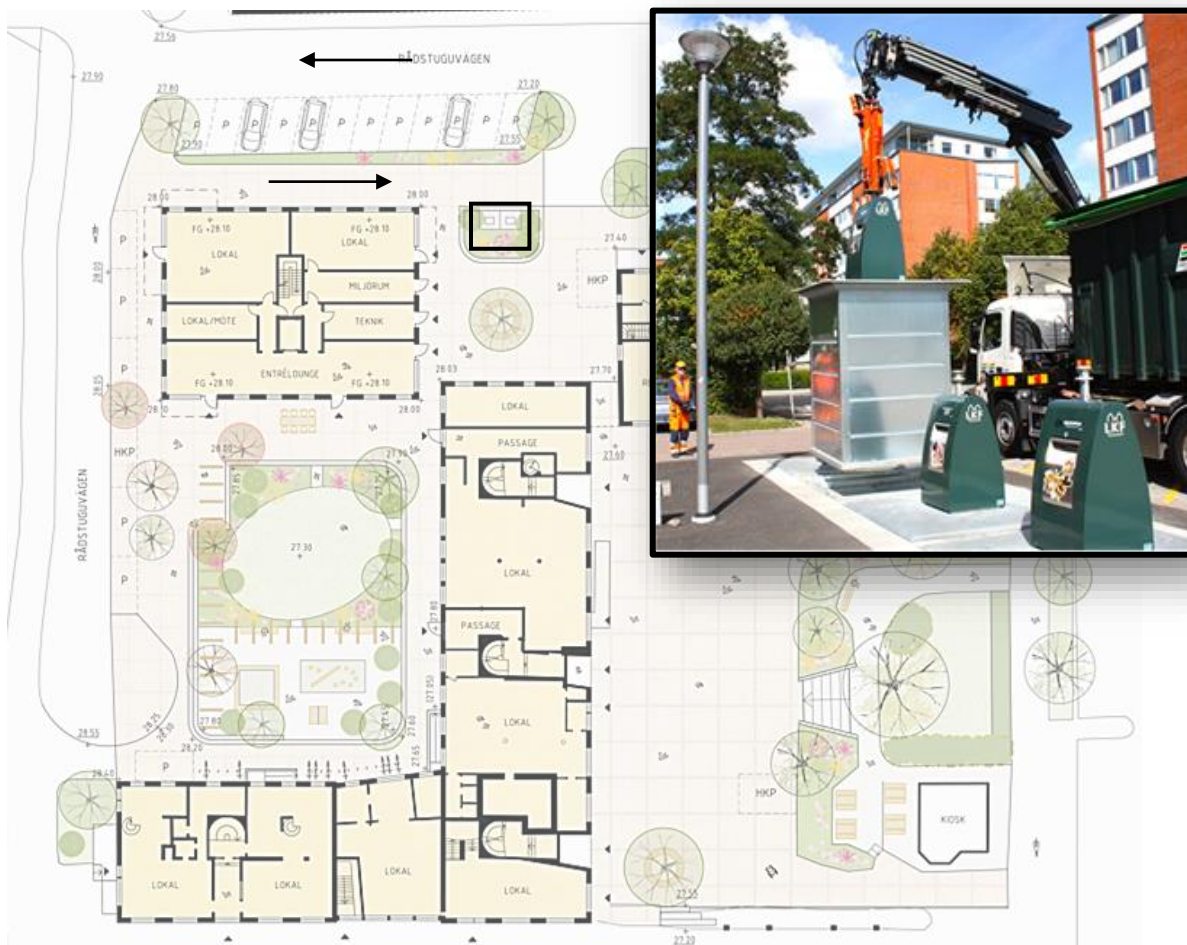
Figur 7. Angöring för sopbil genom avfallshantering med kassuner.
