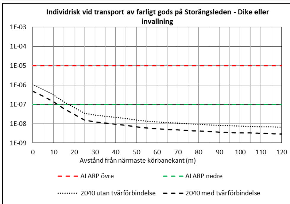
Figur 14. Individrisk längs med Storängsleden givet åtgärden dike i kombination med avåkningsskydd.
