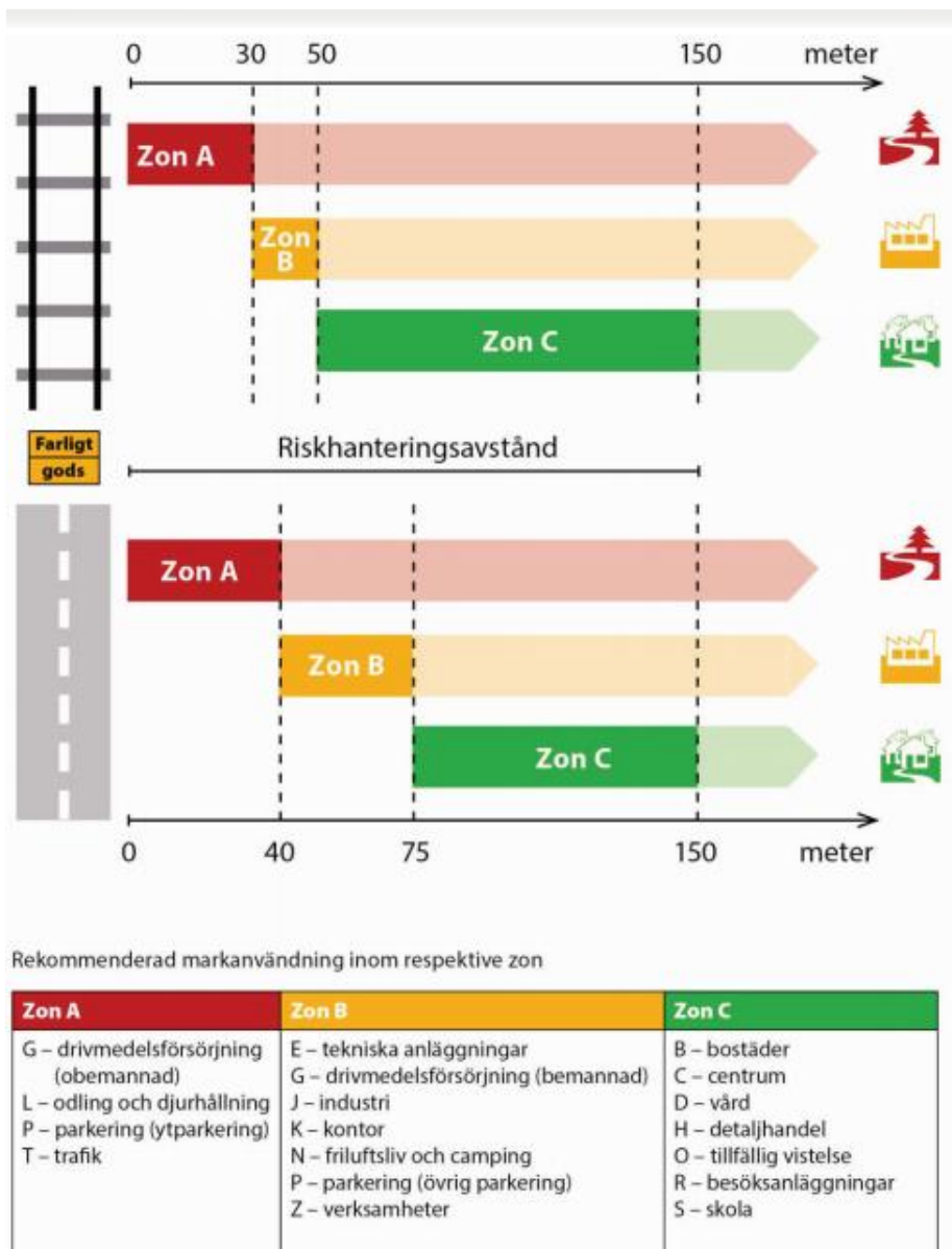
Figur 2. Rekommenderade skyddsavstånd mellan transportleder för farligt gods (väg och järnväg) och olika typer av markanvändning [7]. Avstånden mäts från närmaste vägkant respektive närmaste spårmitte.
