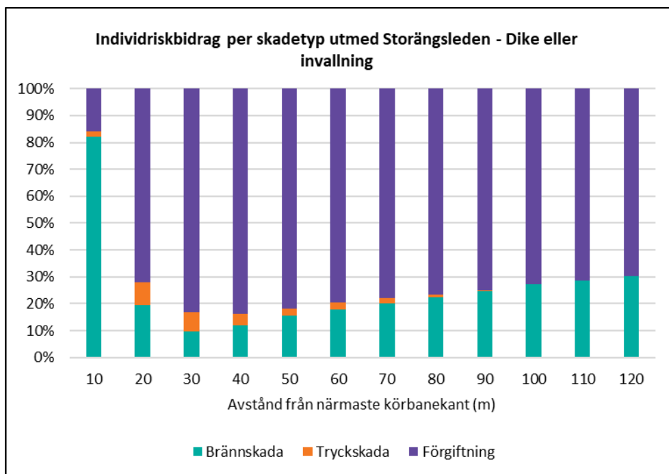
Figur 15. Individriskbidrag från olika skadetyper utmed Storängsleden, givet åtgärden dike i kombination med avåkningsskydd.
