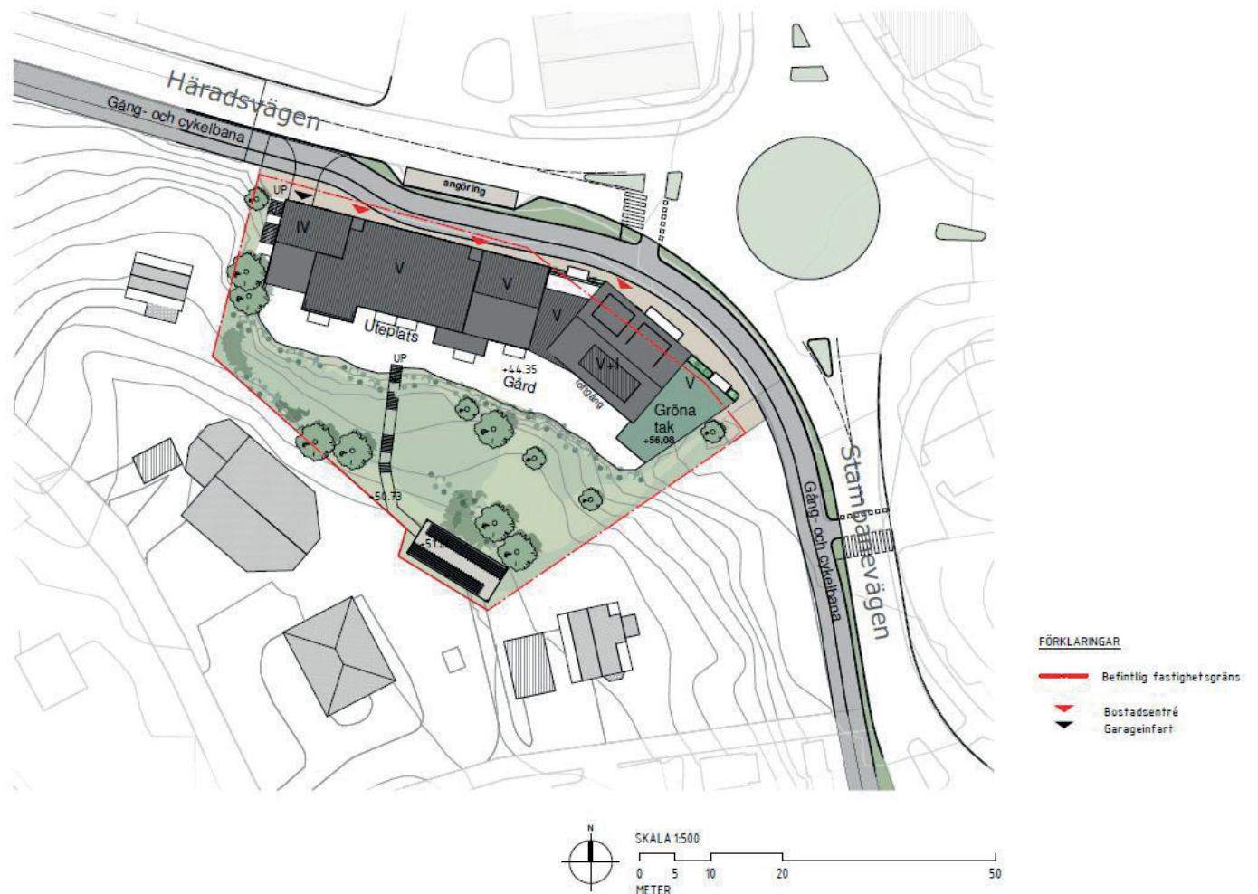
Planförslag avseende fastigheterna Odin 3 och 6.
