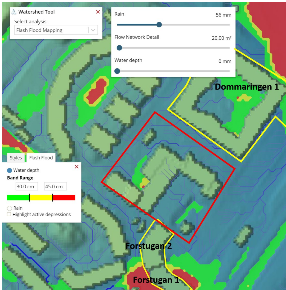
Figur 15 Maximalt vattendjup och flödesvägar vid 56 mm regn vid befintlig situation. Kartan skapades med Scalgo Live (2020). Planområdets gräns markeras med röd linje.
