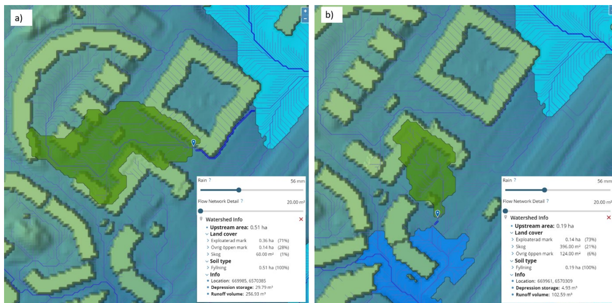
Figur 14 Uppströms avrinningsområde som bidrar till översvämning av planområdet samt nedströms planområdet. Kartan skapades med Scalgo Live (2020).
