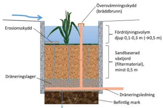
Figur 21 Nedsänkt växtbädd. Bildkälla: Stockholm Vatten och Avfall, 2017a.
