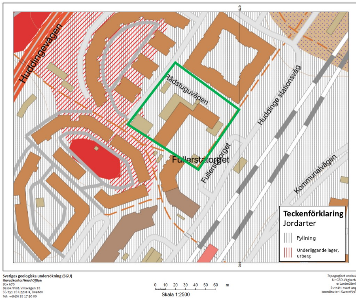
Figur 9 Jordartskarta från SGU med ungefärlig placering av planområdet markerat med grön linje. De grå lodräta linjerna visar fyllning och de röda diagonala linjerna anger att underliggande lager är urberg. (Bildkälla: SGU, 2020a)
