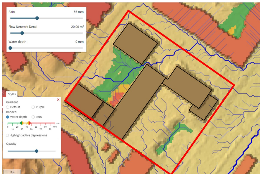
Figur 19 Maximalt vattendjup och flödesvägar vid 56 mm regn. Planerad bebyggelse markeras med fet svart linje och planområdets gräns med röd linje. Figuren visar en situation med planerad bebyggelse där befintliga marknivåer inte förändras. Kartan skapades med ScalgoLive (2022).
