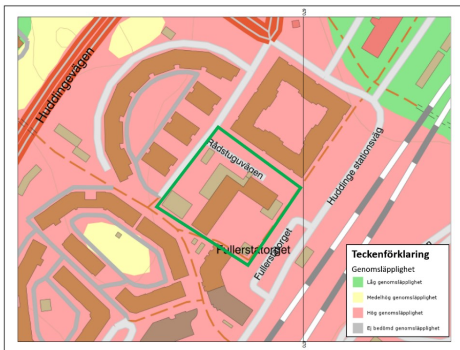
Figur 10 Genomsläpplighetskarta från SGU med ungefärlig placering av planområdet markerat i grönt. De gröna områdena visar låg genomsläpplighet, de gula områdena visar medelhög genomsläpplighet och de röda områdena visar hög genomsläpplighet (Bildkälla: SGU, 2020b)
