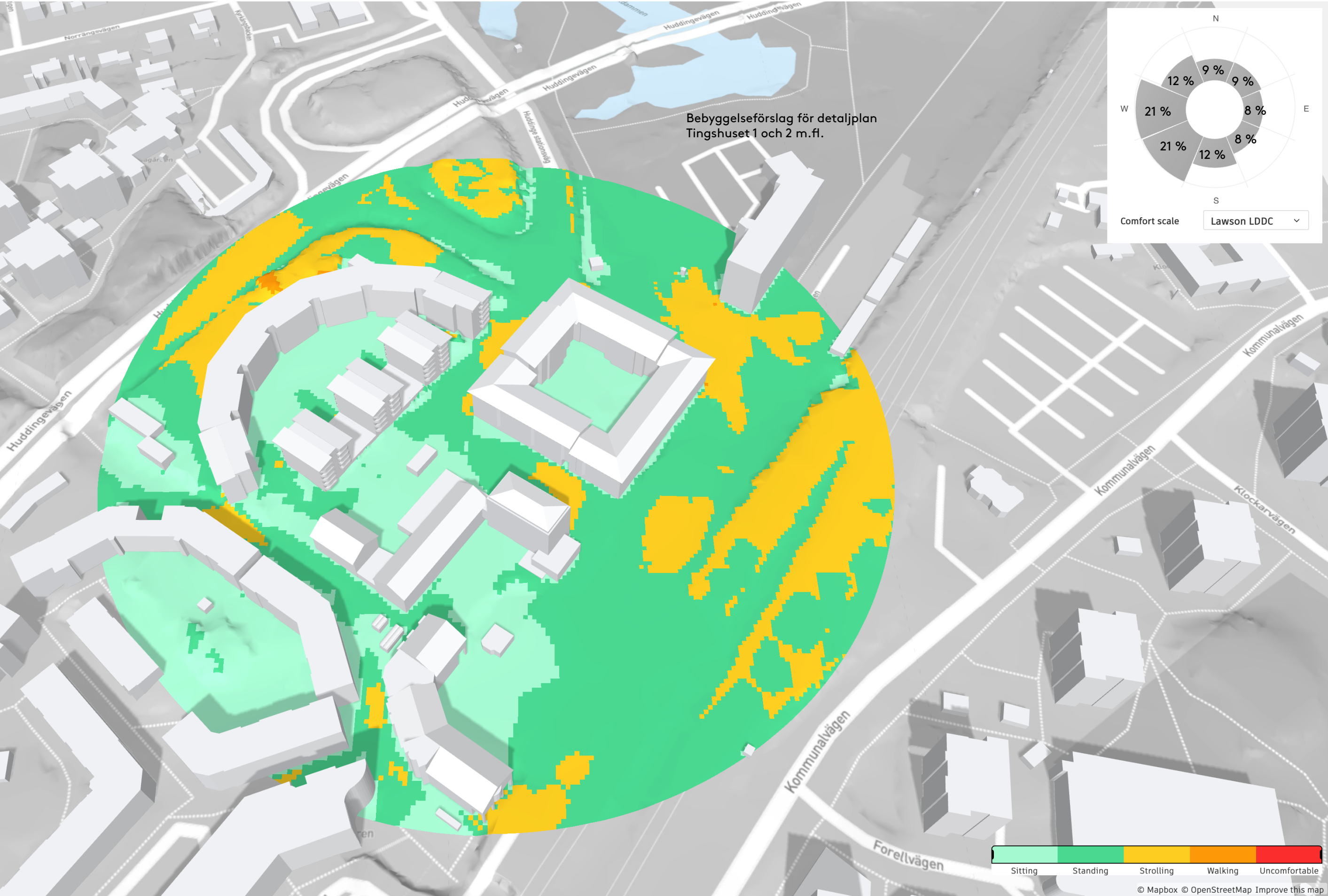
Vindstudie Fullesta torg och Udden 8 - utan förtätningsförslag. Bild visar en vindkomfortanalys för fotgängare 1,75 m över marken. Komfortskalan indikerar var det med största sannolikhet är bekvämt för olika aktivitetsnivåer under längre tidsperioder.
