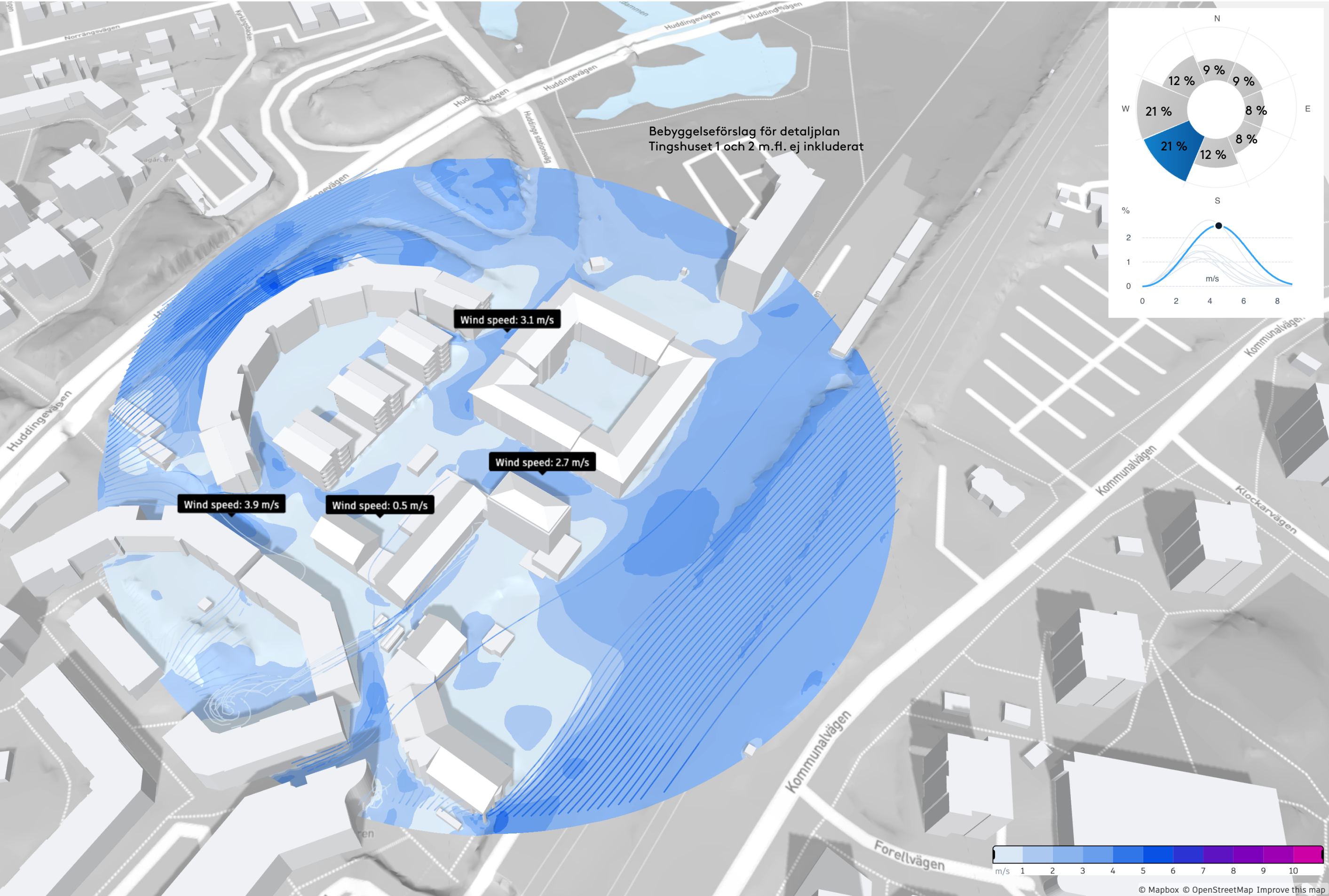
Vindflöde Fullesta torg och Udden 8 - utan förtätningsförslag. Bild visar flödesmönster och medelvind vid vanligast förekommande vindriktning (SV, 21%).
