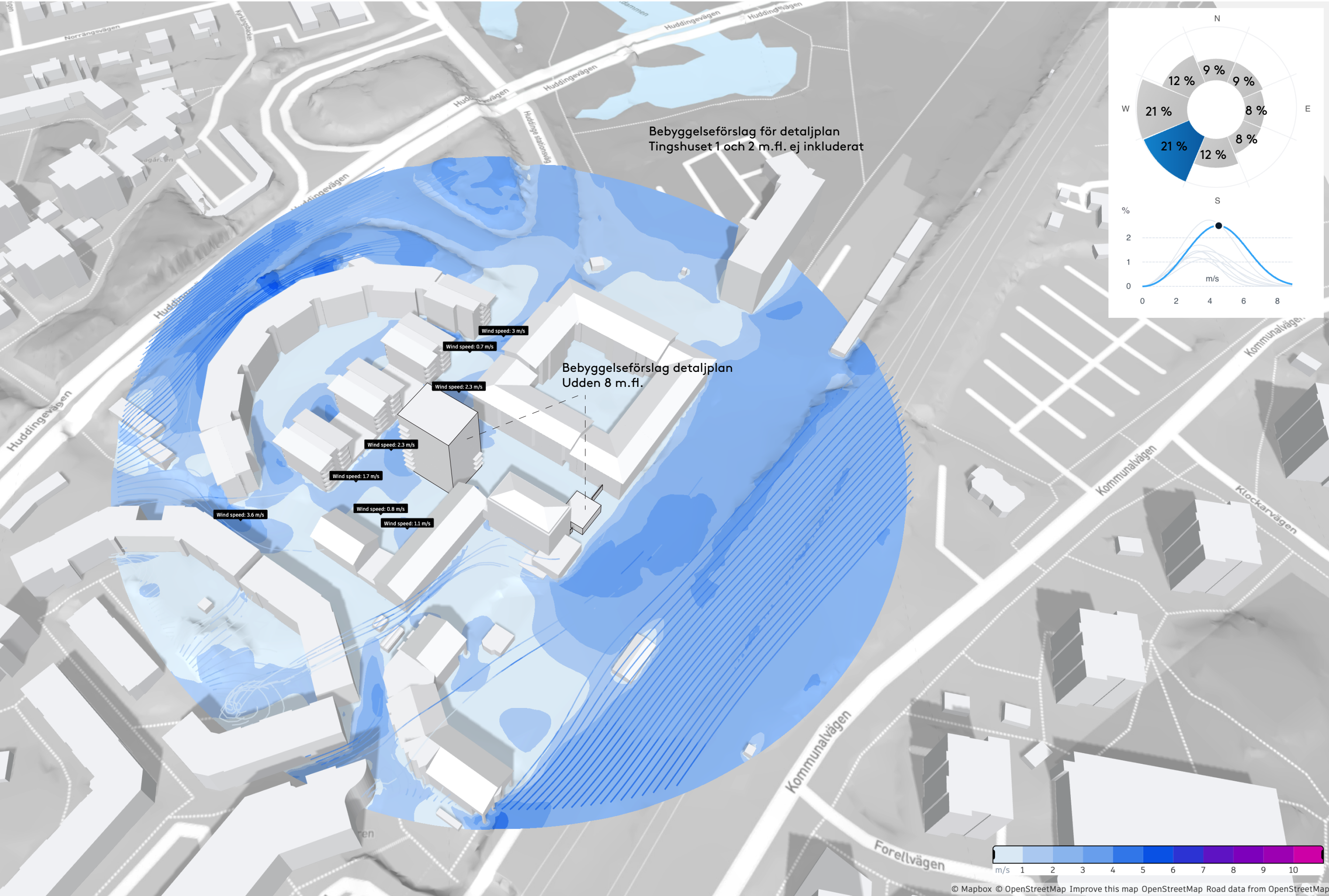
Vindflöde Fullesta torg och Udden 8 - med förtätningsförslag. Bild visar flödesmönster och medelvind vid vanligast förekommande vindriktning (SV, 21%).
