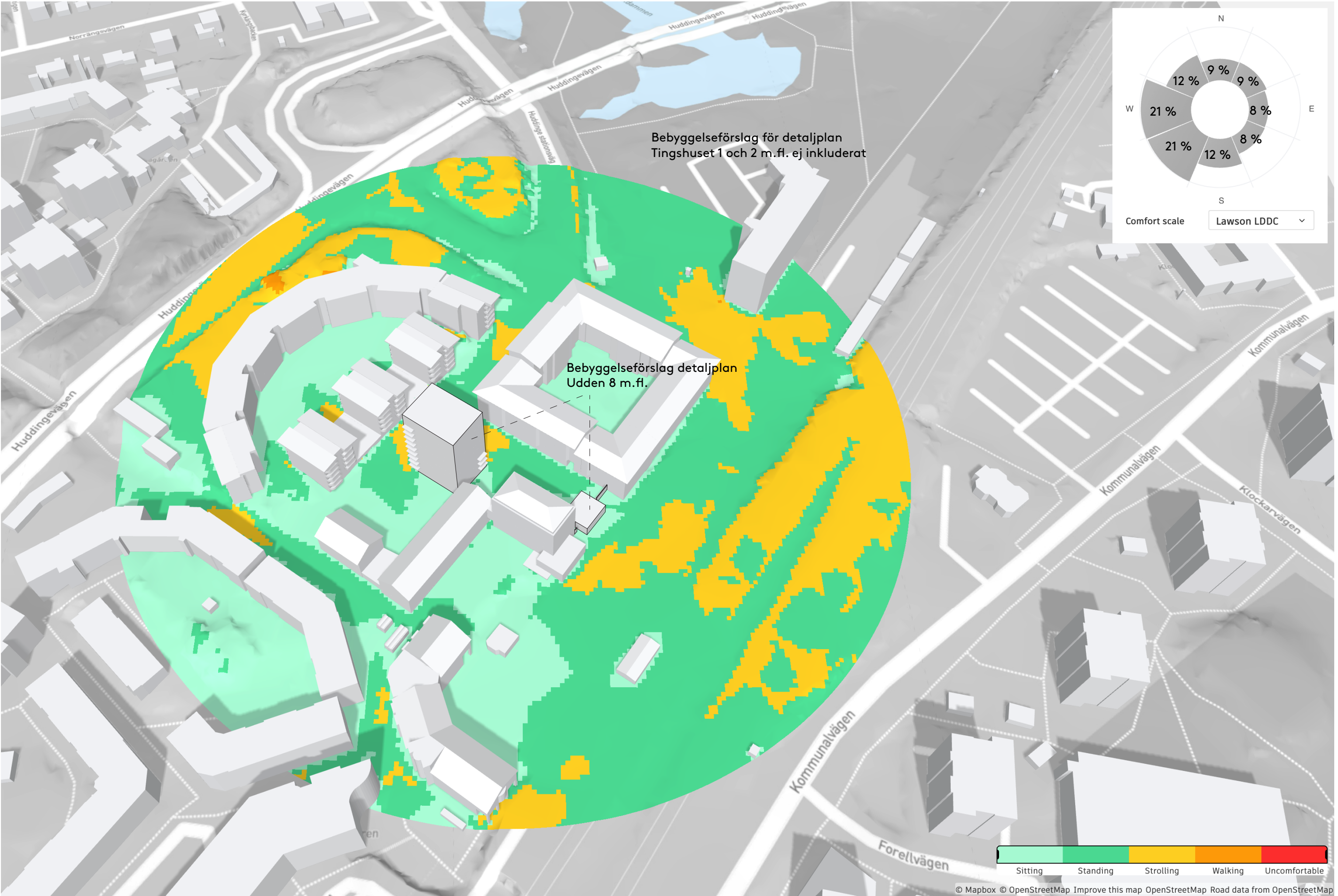
Vindstudie Fullesta torg och Udden 8 - med förtätningsförslag. Bild visar en vindkomfortanalys för fotgängare 1,75 m över marken. Komfortskalan indikerar var det med största sannolikhet är bekvämt för olika aktivitetsnivåer under längre tidsperioder.
