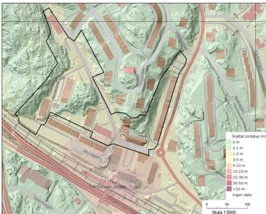
Figur 5 Generaliserad jorddjupskarta med topografisk terrängskuggning. Detaljplaneområdet markerat med svart linje. Källa © SGU.
