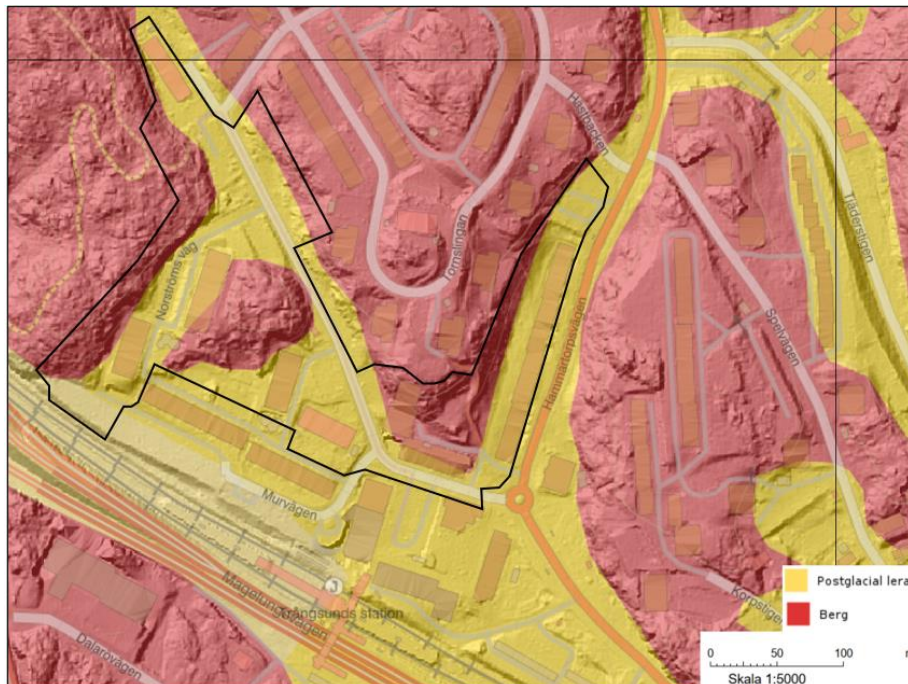
Figur 4 Generaliserad jordartskarta med topografisk terrängskuggning. Detaljplaneområdet markerat med svart linje. Källa © SGU
