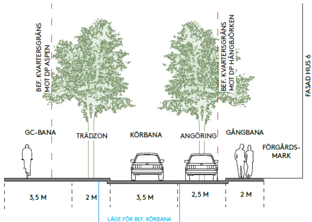
Figur 12. Föreslagen sektion Apelvägen (ÅWL arkitekter)
