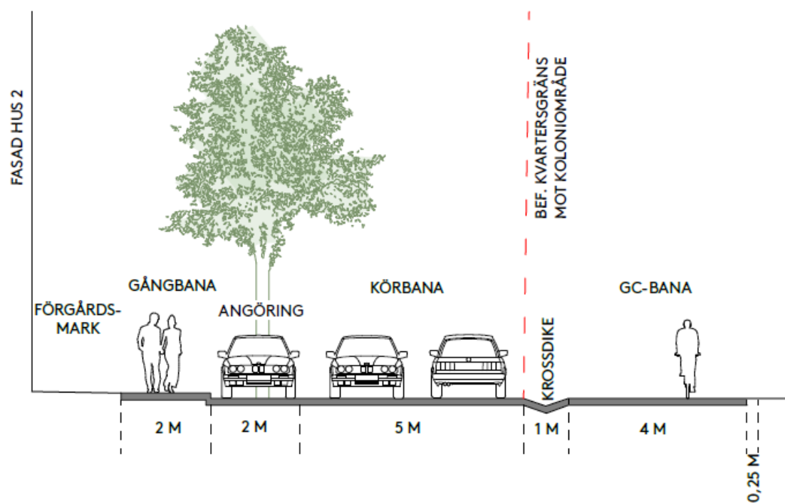
Figur 13. Föreslagen sektion nya angöringsgatan i nordost (ÅWL arkitekter)
