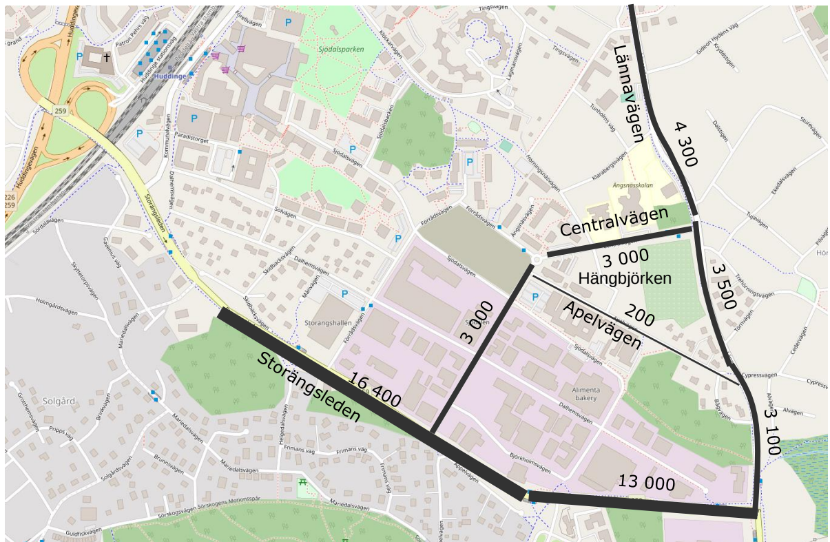
Figur 9. Trafikmängder, årsdygnstrafik, nuläge (mätningarna från de senaste 10 åren)
