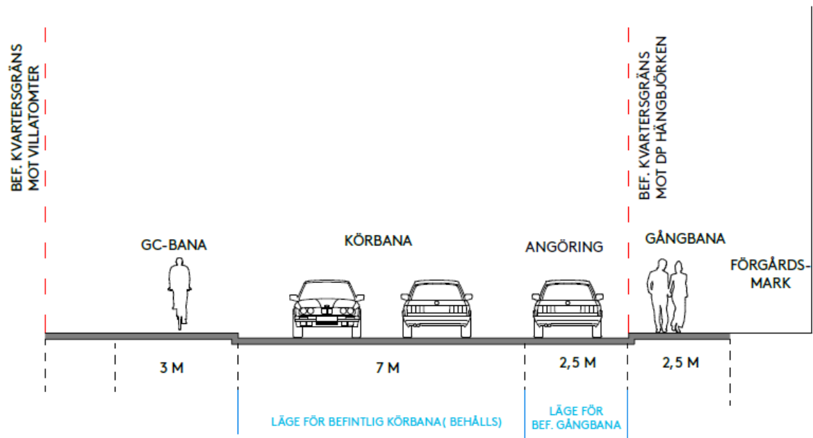
Figur 11. Föreslagen sektion Centralvägen (ÅWL arkitekter)
