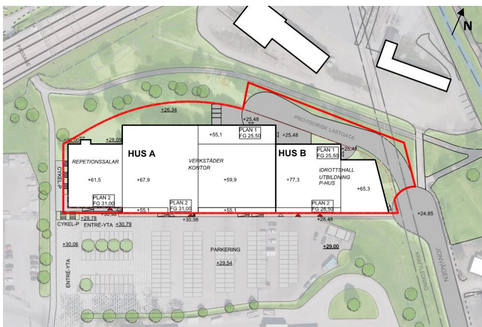
Figur 2.2. Situationsplan Skede 1, gränsen för planområdet är rödmarkerad (Strategisk arkitektur, 2020-05-18).
