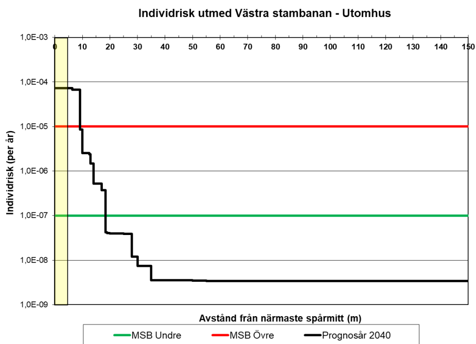
Figur 4.1. Individrisk för oskyddad person utomhus som funktion av avståndet från Västra stambanan (mätt från närmaste spårmit efter utbyggnad).
