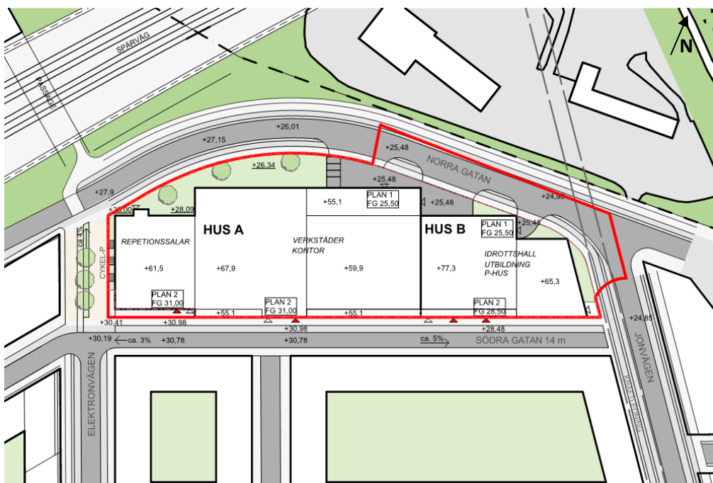
Figur 2.3. Situationsplan Skede 2, gränsen för planområdet är rödmarkerad (Strategisk arkitektur, 2020-05-18).
