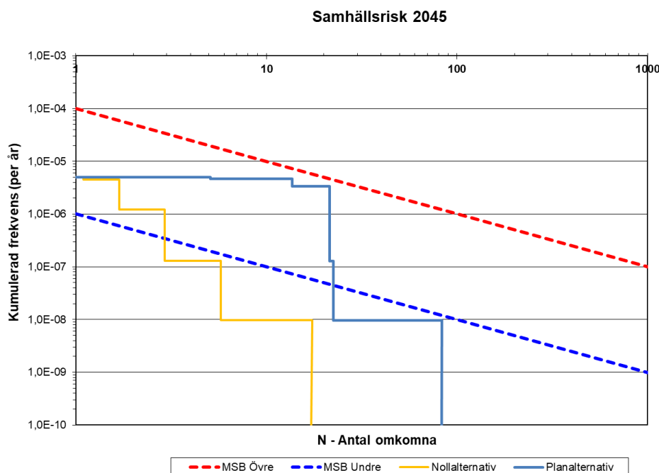
Figur 5.3. F/N-kurva som redovisar samhällsrisknivån för planområdet och dess närmaste omgivning med avseende på olycksrisker förknippade med E4/E20 Södertäljevägen inklusive ramp. (Observera att frekvens och konsekvens redovisas med logaritmisk skala.)
