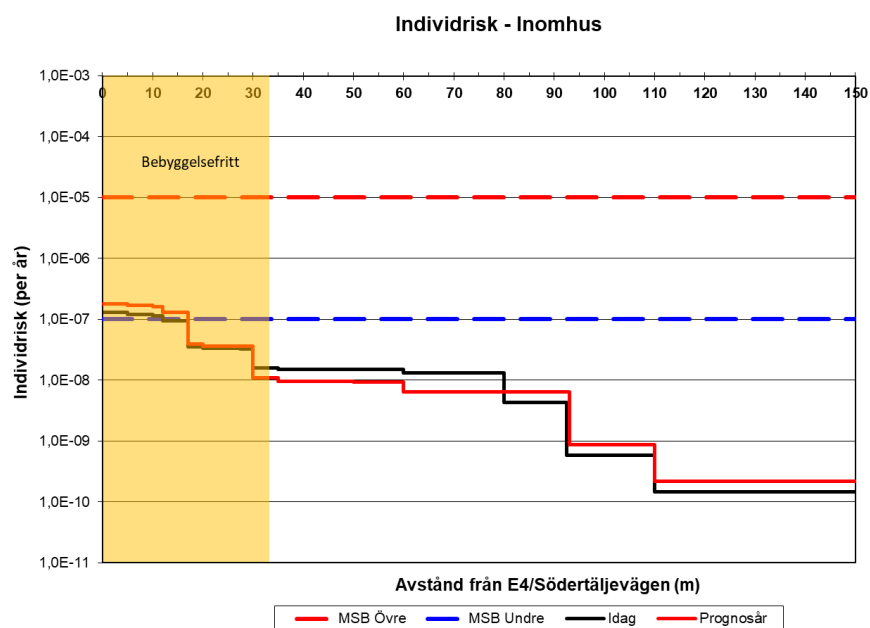
Figur 5.2. Individrisk inomhus utmed E4/E20 Södertäljevägen. Markerat avstånd till bebyggelsefritt avser avstånd från väggkant E4/E20 till byggnader med stadigvarande verksamhet (dvs. ej båtförvaring). (Observera att frekvensen redovisas med logaritmisk skala.)
