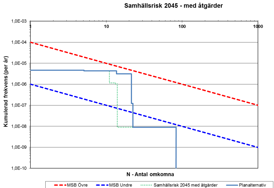
Figur 6.1. Samhällsrisk med åtgärder.
