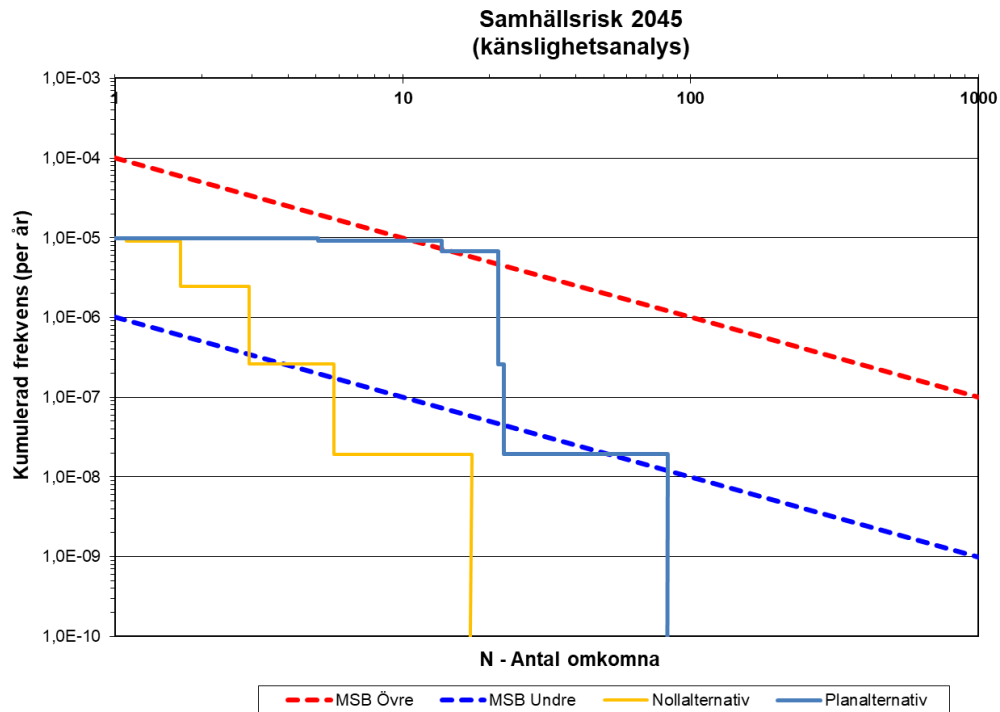
Figur C. 6. Känslighetsanalys – Samhällsrisk. (Observera att frekvens och konsekvens redovisas med logaritmisk skala).
