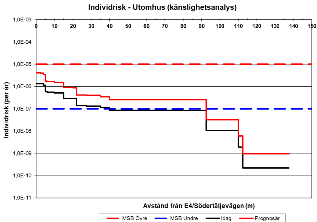
Figur C.4. Känslighetsanalys – individrisk utomhus. (Observera att frekvensen redovisas med logaritmisk skala).
