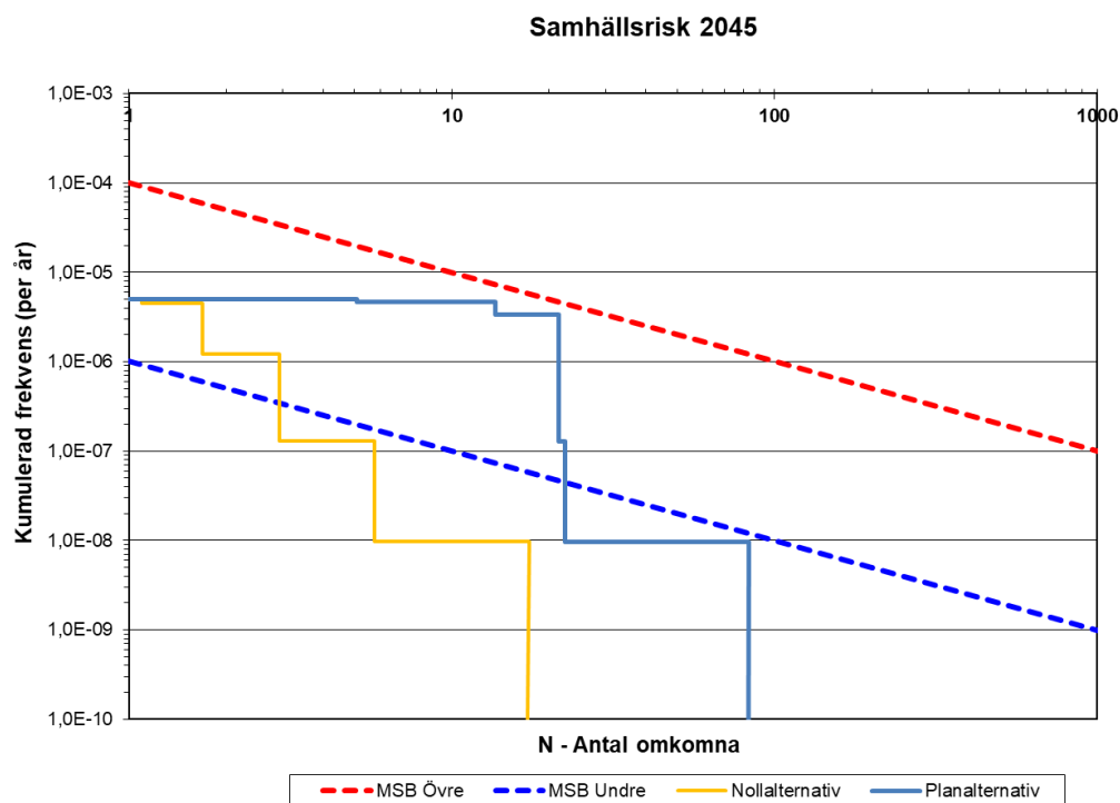
Figur C.3. F/N-kurva som redovisar samhällsrisknivån för planområdet samt kringliggande bebyggelse med avseende på olycksrisker förknippade med E4/E20 Södertäljevägen inklusive ramp som förbinder vägen med Tvärförbindelse Södertörn. (Observera att frekvens och konsekvens redovisas med logaritmisk skala).
