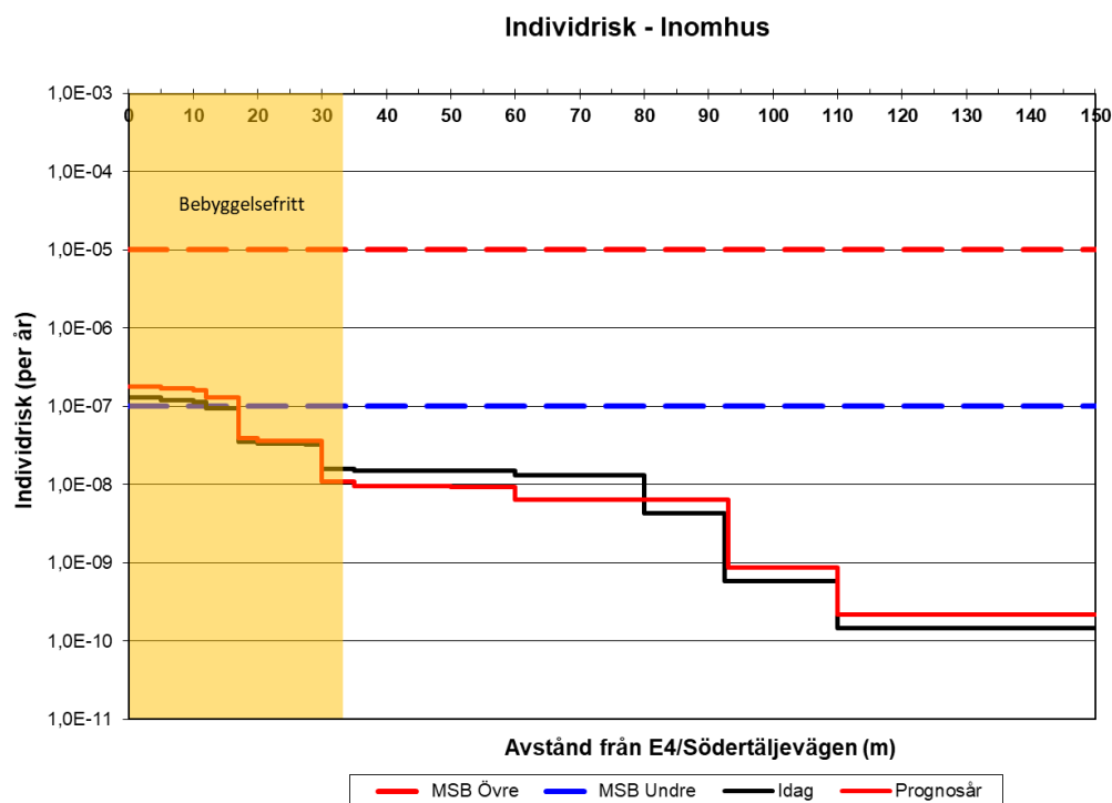
Figur C. 2. Individriskprofiler för person inomhus inom planområdet som funktion av avståndet till E4/E20 Södertäljevägen inkl. ramp. Det bebyggelsefria avståndet till E4/E20 är markerat i figuren. (Observera att frekvensen redovisas med logaritmisk skala).
