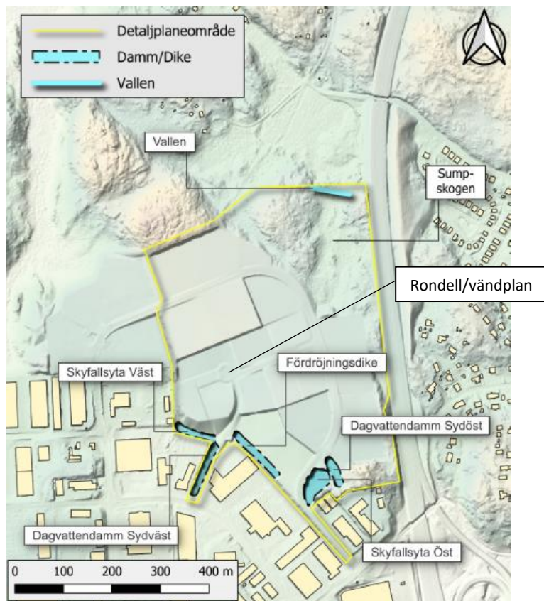
Figur 15-4 Skyfallsåtgärder inom planområdet.
