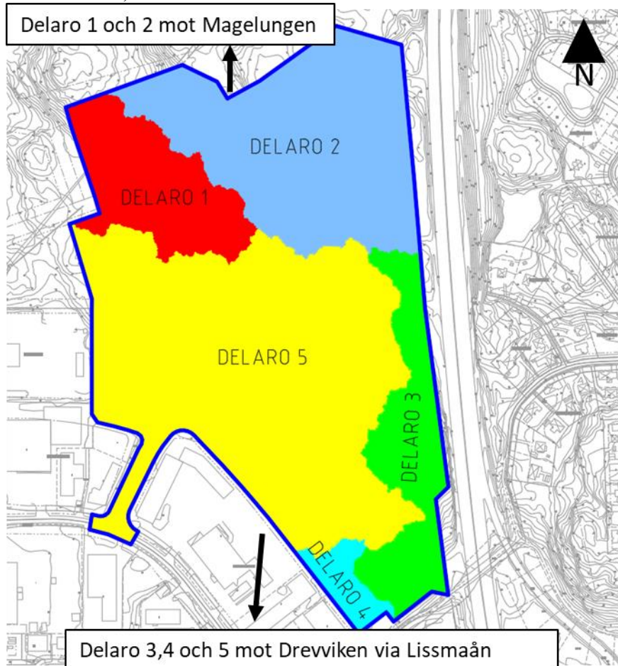
Figur 5-1. Delavrinningsområden för ytlig avrinning utifrån befintlig situation.
