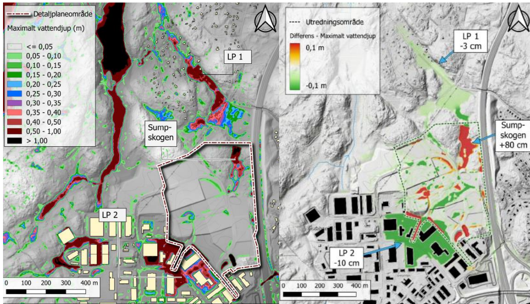
Figur 15-5 Till vänster: Maximalt vattendjup för ett 100-årsregn (med klimatafaktor 1,25) efter utbyggnad. Till höger: Differens mellan nuläget och planförslaget. Grönt innebär en minskning av vattendjupen. (Rejlers, 2025)
