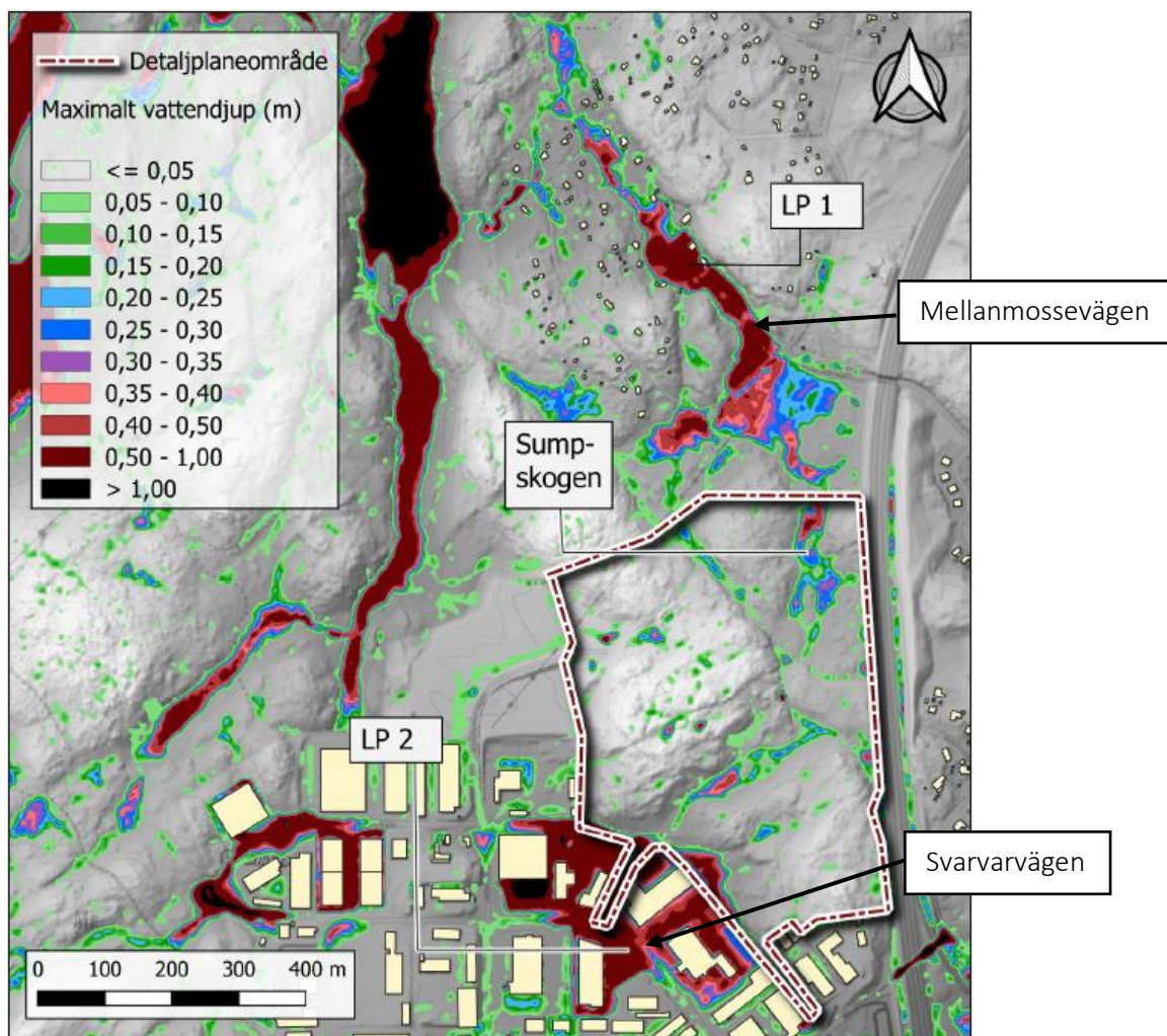
Figur 8-3 Skyfallskartering för 100-årsregn (inklusive klimatafaktor 1,25), befintlig situation och med etapp 1 färdigställd. (Rejlers, 2025).
