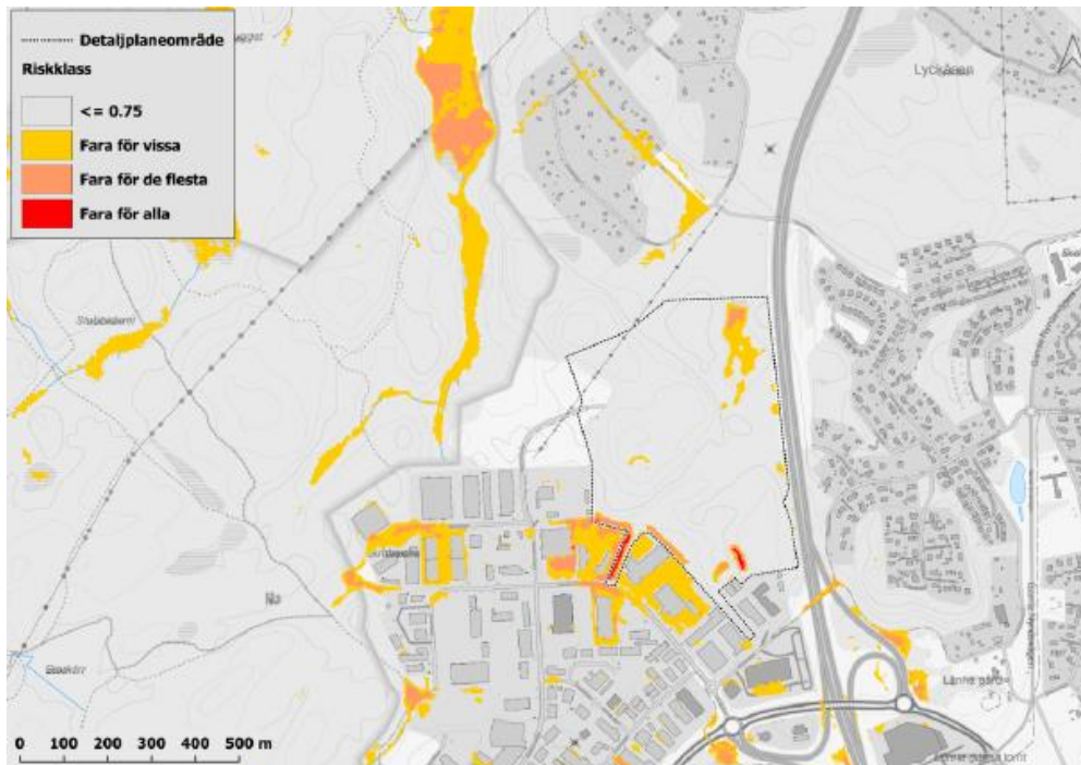
Figur 15-6 Klassning av risker för människor i samband med översvämningshändelse, med utbyggd detaljplan (Rejlers, 2025).
