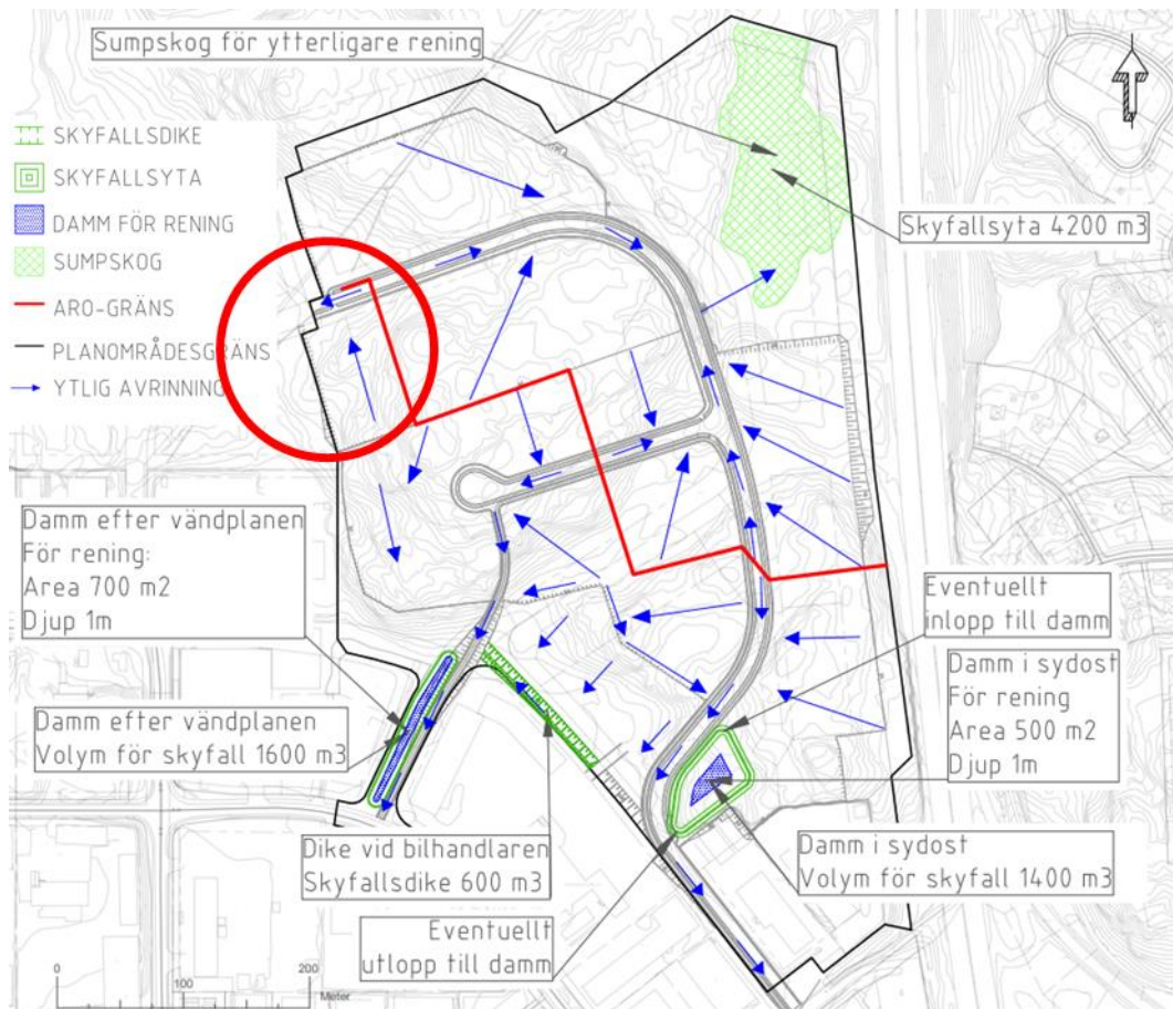
Figur 16-1. Inringat område har antagits kunna ledas till etapp 1 och Drevviken via Lissmåån
