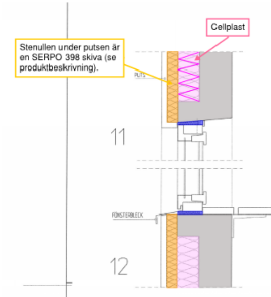
Figur 1. Sektionsprincip över fönster.
