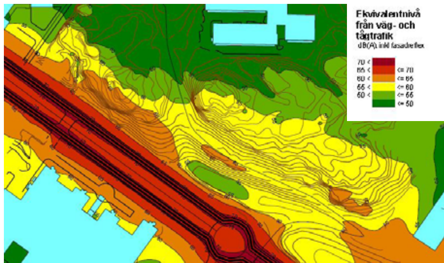
Bullerkartering visar att rekommenderade ljudnivåer riskerar att överstigas, Bullerutredning, Ramböll
