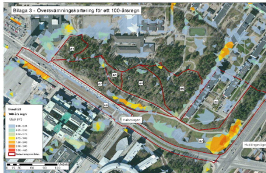
Översvämning vid 100-årsregn, Dagvattenutredning, Atkins.
