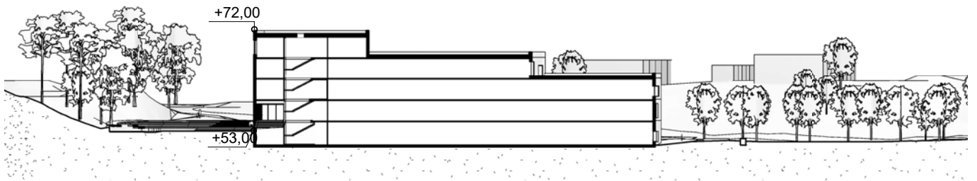
Sektion A-A Genom F-3-flygel sett mot parkering
