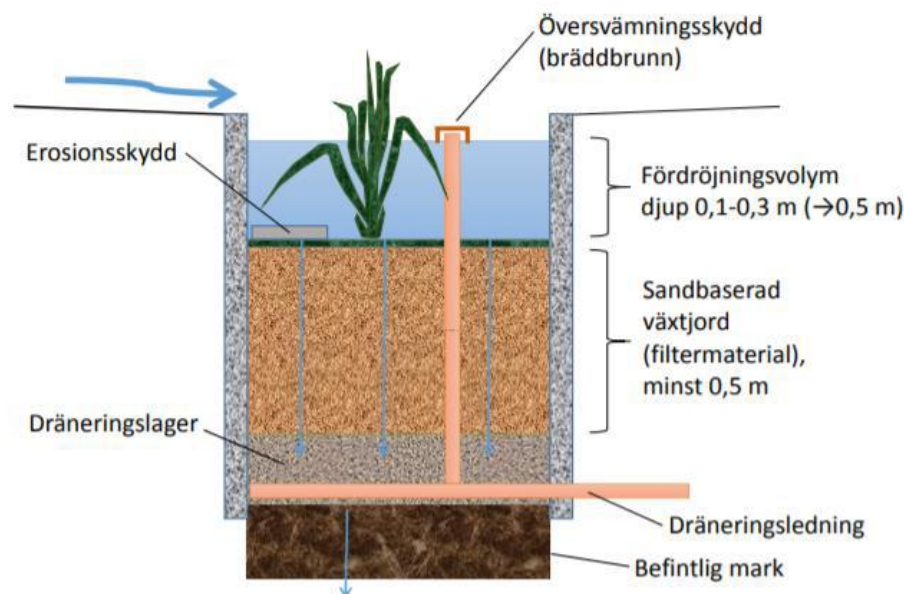
Figur 14. Principskiss på växtbädd. Källa: Stockholm stad, 2018.
