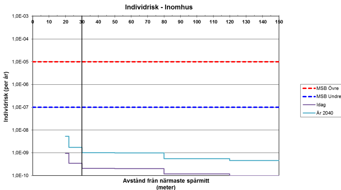
Figur C.2. Individriskprofiler för person inomhus som funktion av avståndet till Nynäsbanan (mätt från närmaste spårmitt). Utan hänsyn tagen till bebyggelse eller andra avskärmande barriärer inom planområdet. Svart markering visar minsta avstånd mellan närmaste spårmitt och byggnad inom planområdet. (Observera att frekvensen redovisas för logaritmisk skala).
