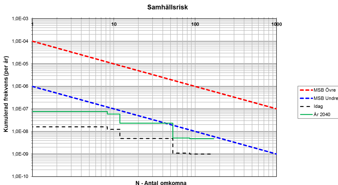
Figur 4.3. F/N-kurva som redovisar samhällsrisknivån för planområdet och dess närmaste omgivning med avseende på olycksrisker förknippade med Nynäsbanan.
