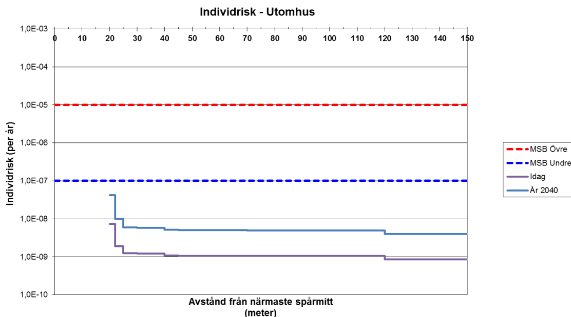
Figur C.1. Individriskprofiler för oskyddad person utomhus som funktion av avståndet till Nynäsbanan (mätt från närmaste spårmitt). Utan hänsyn tagen till bebyggelse eller andra avskärmande barriärer inom planområdet. (Observera att frekvensen redovisas för logaritmisk skala).
