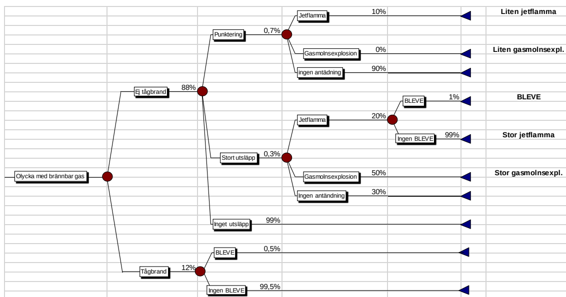
Figur A.2. Händelsetråd olycka med transport av brännbar gas (klass 2.1).
