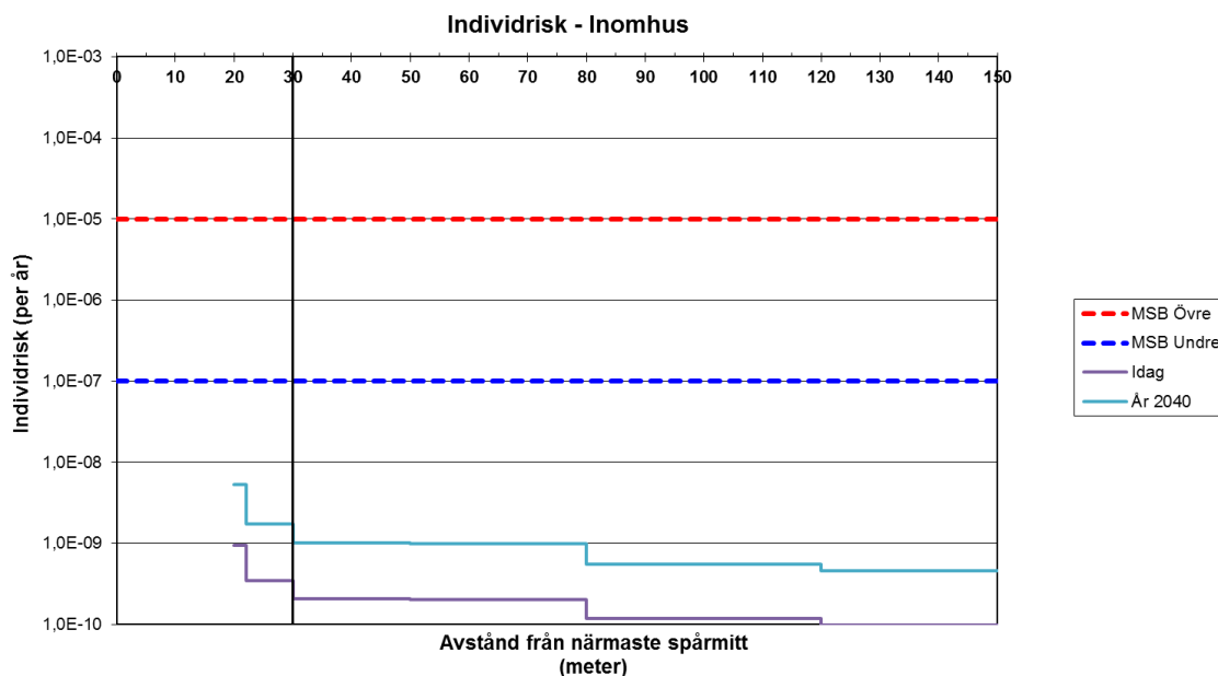
Figur 4.2. Individrisk inomhus utmed Nynäsbanan. Svart markering visar minsta avstånd mellan närmaste spårmitte och byggnad inom planområdet. (Observera att frekvensen redovisas med logaritmisk skala).
