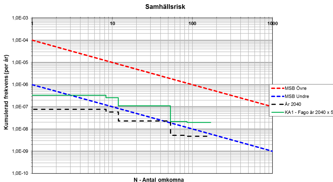
Figur C.4. F/N-kurva som redovisar samhällsrisknivån för planområdet samt kringliggande bebyggelse med avseende på olycksrisker förknippade med Nynäsbanan. (Observera att frekvens och konsekvens redovisas med logaritmisk skala).
