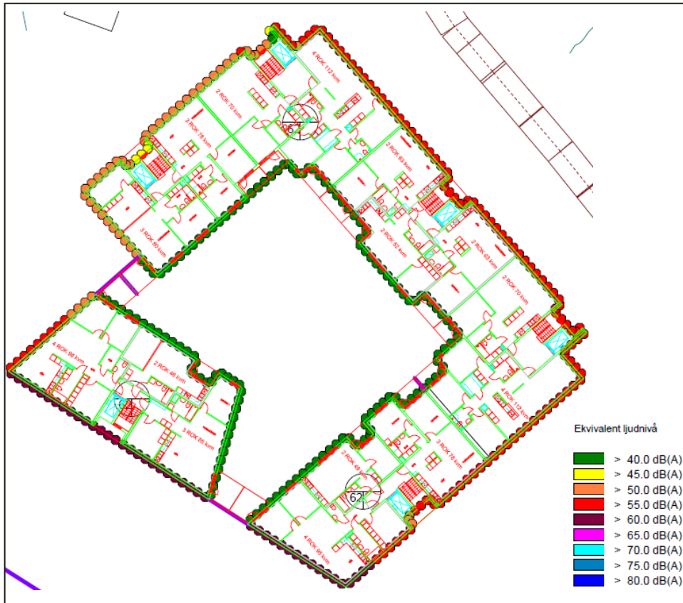
Ekvivalent ljudnivå samlat buller väg – och spårtrafik
