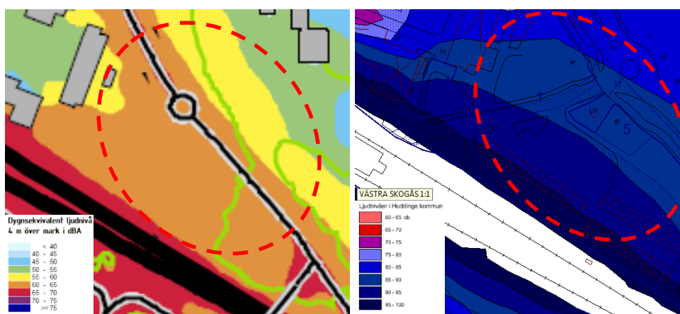
Dygnsekvivalent ljudnivå väg och spår 4 m över mark, bilden till vänster och maximala ljudnivåer järnväg 4 m över mark (Tyrens 2012), bilden till höger.
