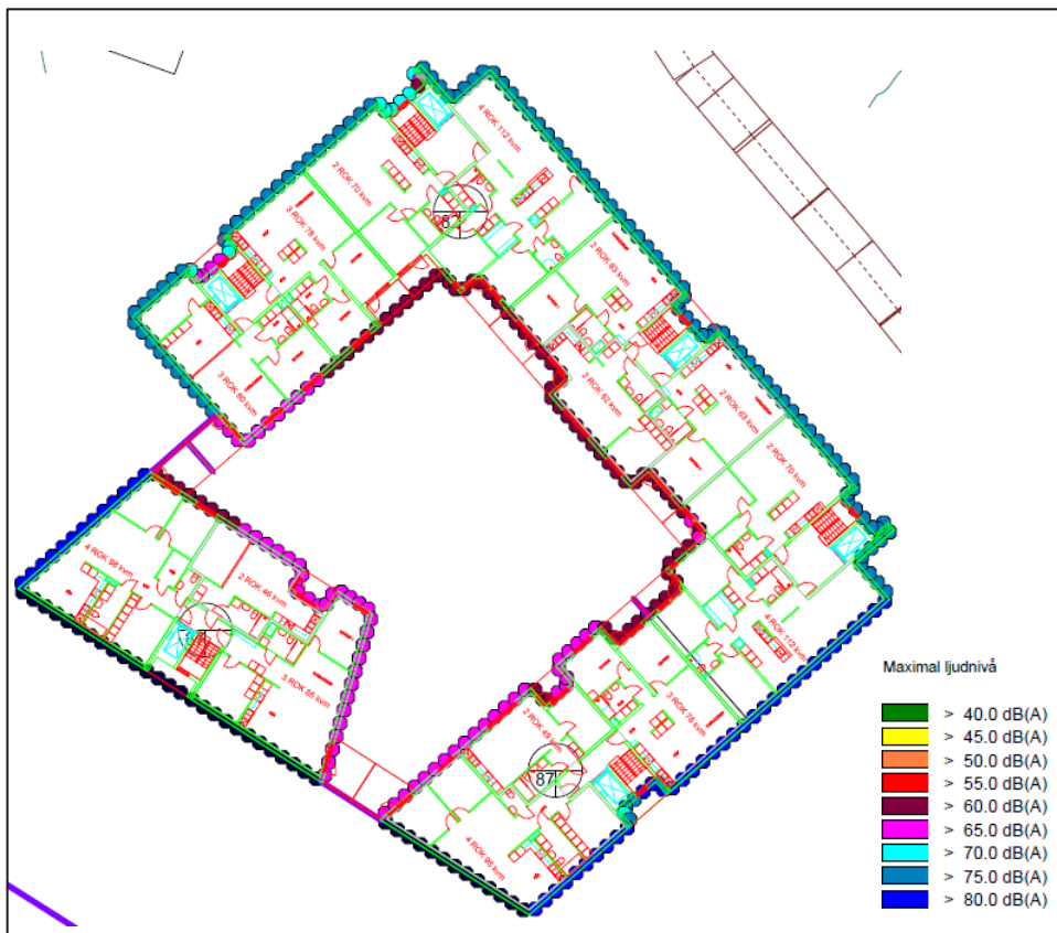
Maximal ljudnivå samlat buller väg- och spårtrafik
