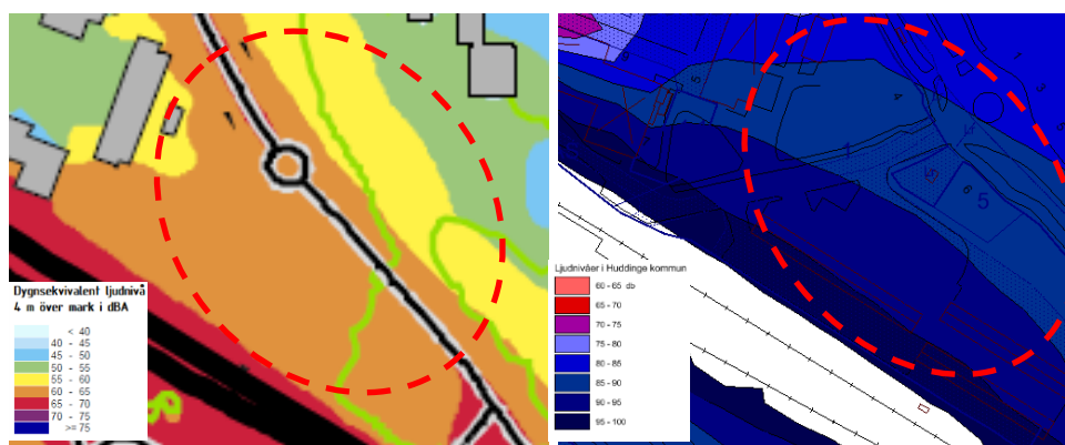
Dygnsekvivalent ljudnivå väg och spår 4 m över mark, bilden till vänster och maximala ljudnivåer järnväg 4 m över mark (Tyréns 2012), bilden till höger.
